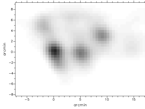
NGC6822
