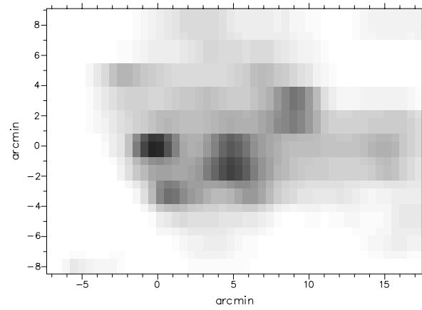
NGC 6822
