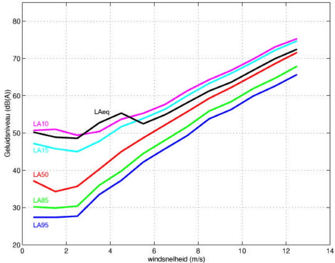
Figuur 3.4: lijngrafieken van een aantal percentie niveaus en het equivalente geluidsniveau uitgezet tegen de windsnelheid
