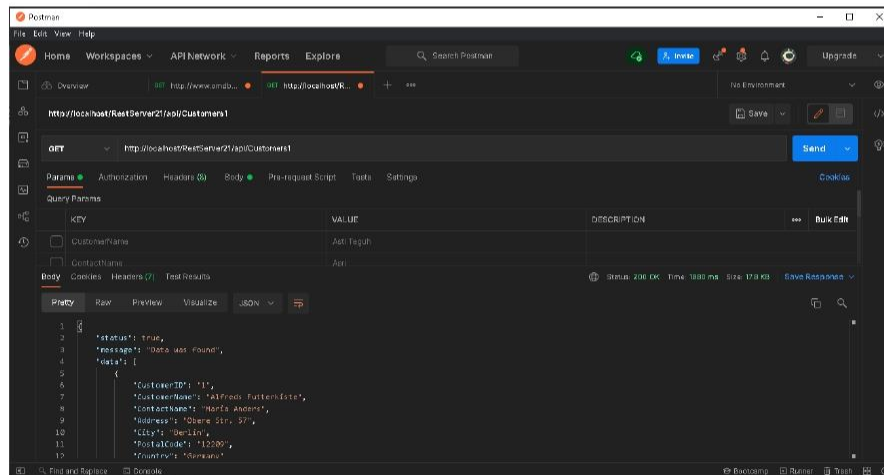
Gambar 10. Request method GET dari rest server dengan aplikasi Postman
