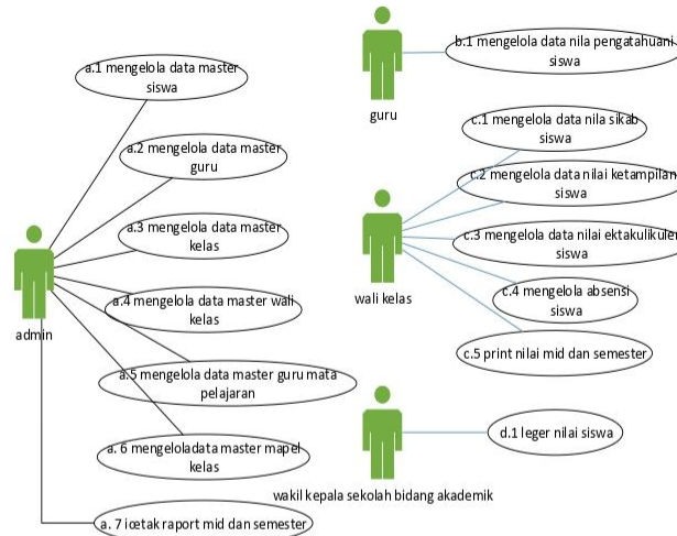
Gambar 3. Use Case Diagram Aplikasi Penilaian Siswa
