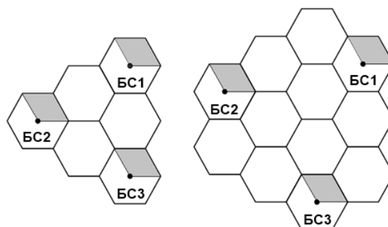
Рис. 2. Сценарии моделирования для оценки SNIR на входе приемника АС для различной размерности кластера N частотного планирования
