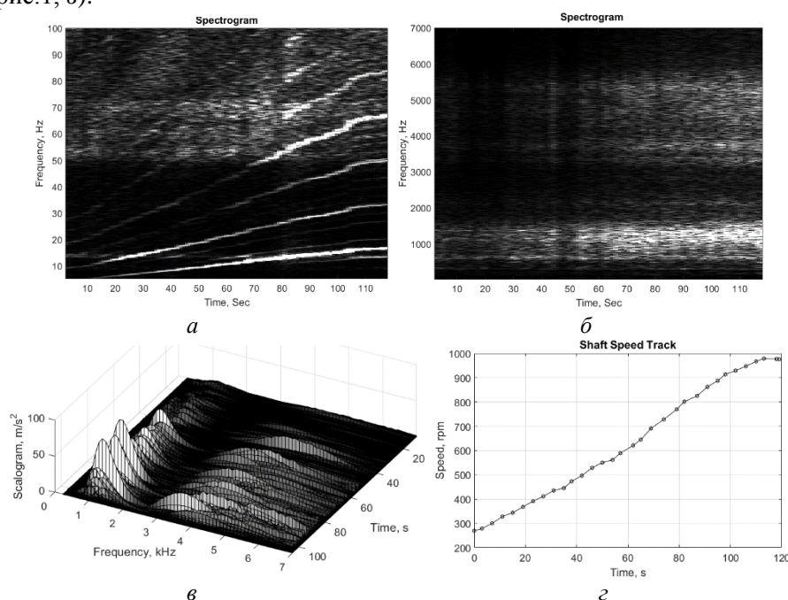
Рис. 1. Частотно-временное представление нестационарного сигнала:
