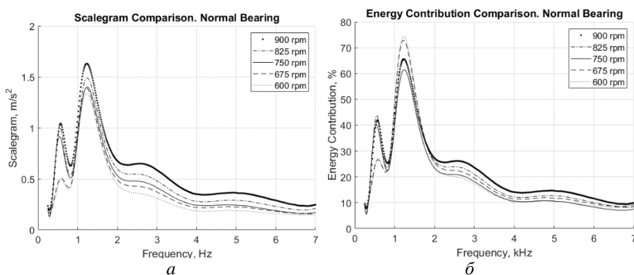
Рис. 3. Нормальный подшипник при различных скоростях вращения: a – скейлограмма; б – энергетический вклад
