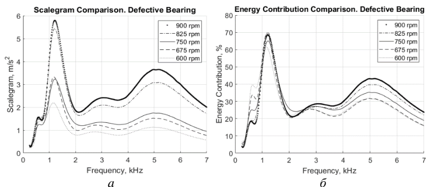
Рис. 2. Дефектный подшипник при различных скоростях вращения: a – скейлограмма, б – энергетический вклад
