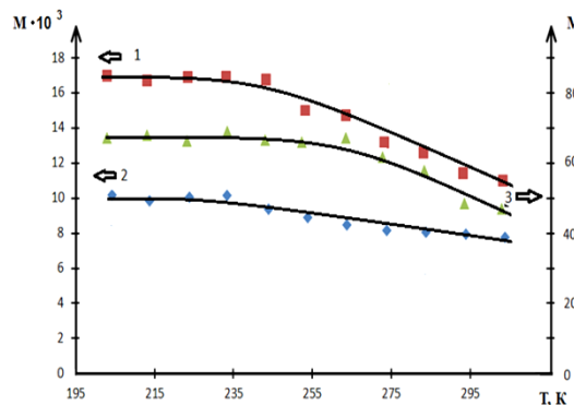
Рис. 3. Зависимость коэффициента усиления фототока от температуры: 1 – для структуры p+-p-n+ ; 2 – для структуры n+-n-p+ ; 3 – для лавинного фотодиода
