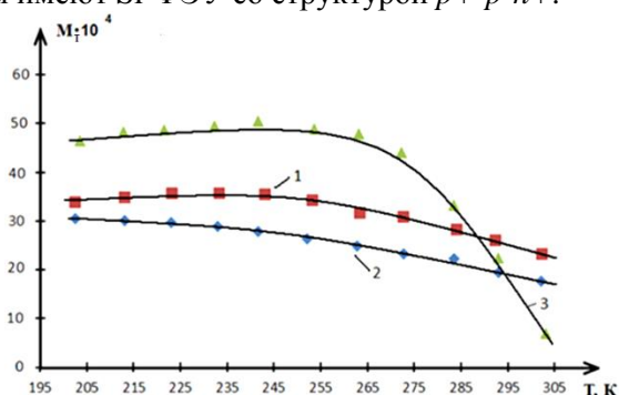
Рис. 2. Зависимость коэффициента усиления темного тока от температуры: 1 – для структуры p+-p-n+ ; 2 – для структуры n+-n-p+ ; 3 – для лавинного фотодиода
