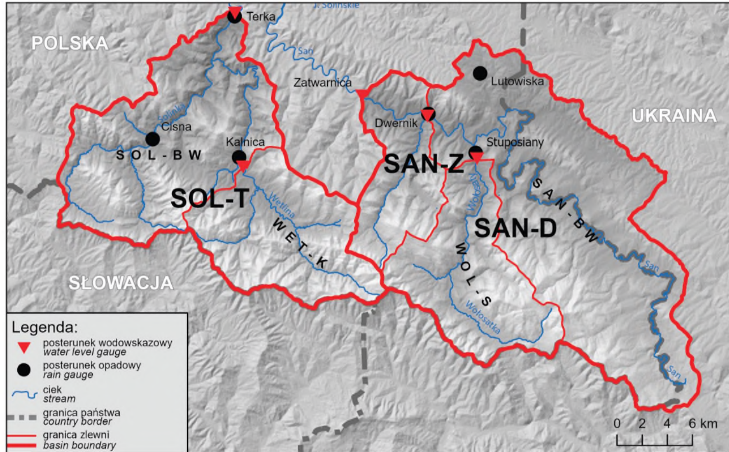
Ryc. 1. Położenie badanych zlewni wraz z lokalizacją posterunków wodowskazowych i opadowych IMGW-PIB. Skróty nazw zlewni wyjaśniono w Tab. 1. Fig. 1. The studied catchments, rainfall and discharge gauging stations (IMGW-PIB). The catchment name abbreviations explained in Table 1.
