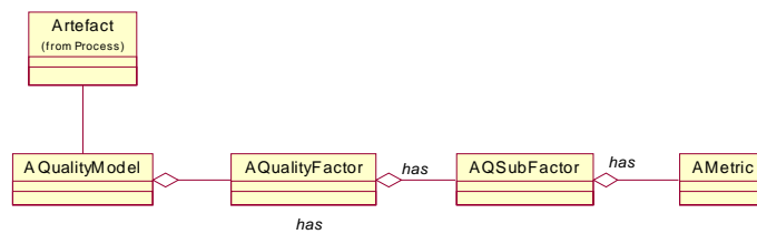
Figura 7. Modelo de calidad para los componentes
