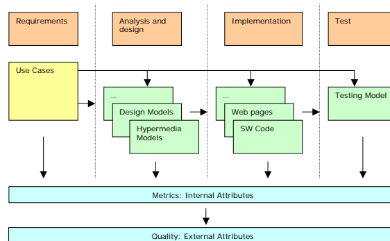
Figura 8. Proceso individual como una instancia del sistema de medidas
