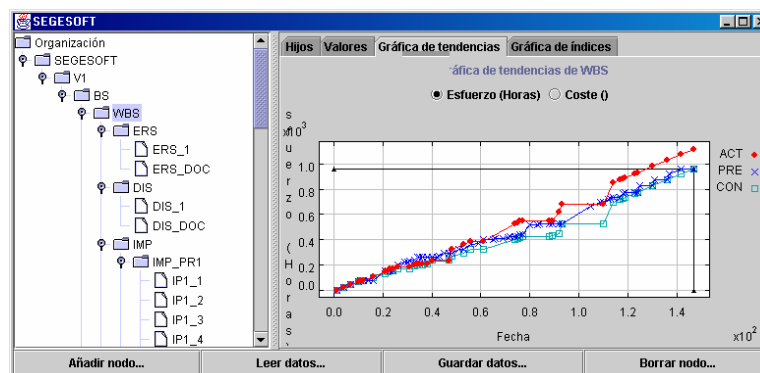
Figura 3. Ejemplo del interfaz gráfico
