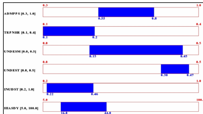
Figura 6. Presentación gráfica de la primera regla
