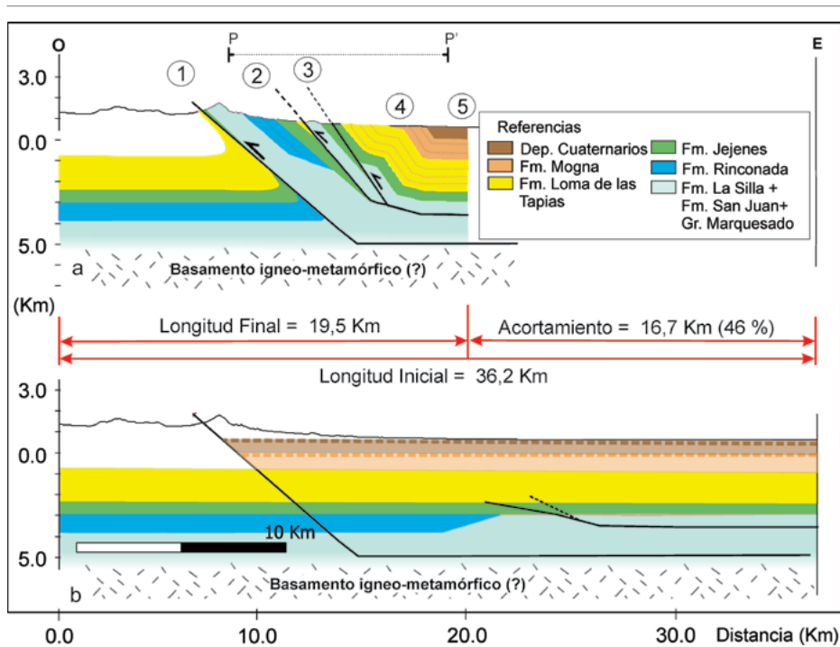
Figura 10. Modelo estructural propuesto para el extremo austral de la falla La Rinconada en la latitud del cerro Piedras de Afilar (ver traza del perfil P-P' en Fig. 3). A) Modelado forward con el software 2D Move en base a observaciones de campo y relaciones estratigráficas y estructurales indicadas en este trabajo. (1) Corrimiento Villicum-Zonda-Pedernal; (2) Falla cerro Piedras de Afilar; (3) Falla La Rinconada; (4) Sinclinal del Este (5) Cerro Valdivia. B) Estado inicial previo a la deformación. Los depósitos cuaternarios y la Formación Mogna aparecen en línea punteada asumiendo que son posteriores al ascenso de la sierra Chica del Zonda, limitada por el corrimiento Villicum Zonda.
