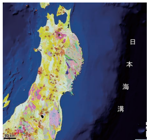
図1 東北地方のシームレス地質図
