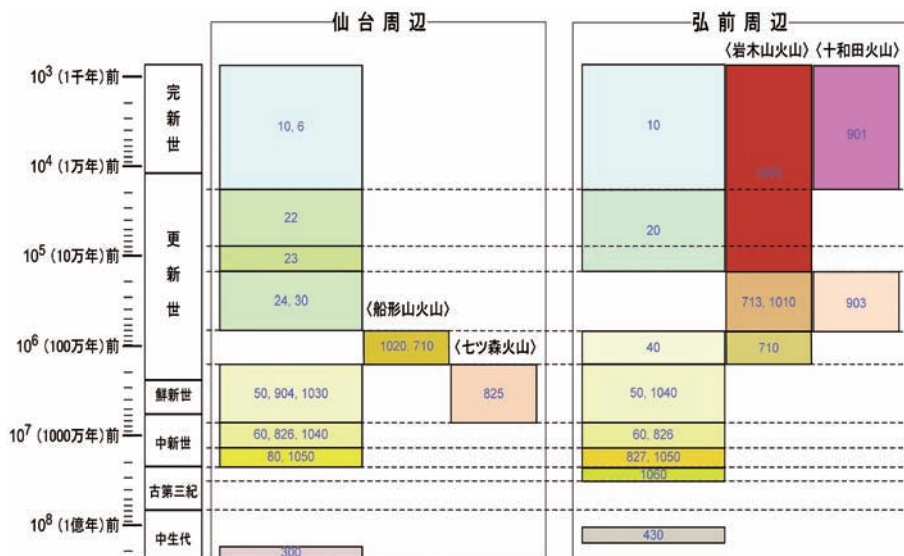
図6 仙台仙台区間地域と弘前区間地域の地質構成の比較
