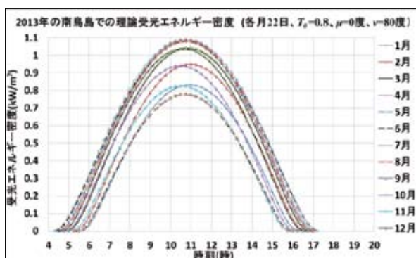
図18 2013年各月22日の受光エネルギー ( \mu = 0 度、 \nu = 80 度、 T_0 = 0.8 )
