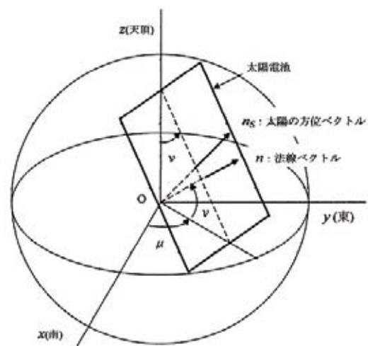
図16 太陽電池の設置と座標系
