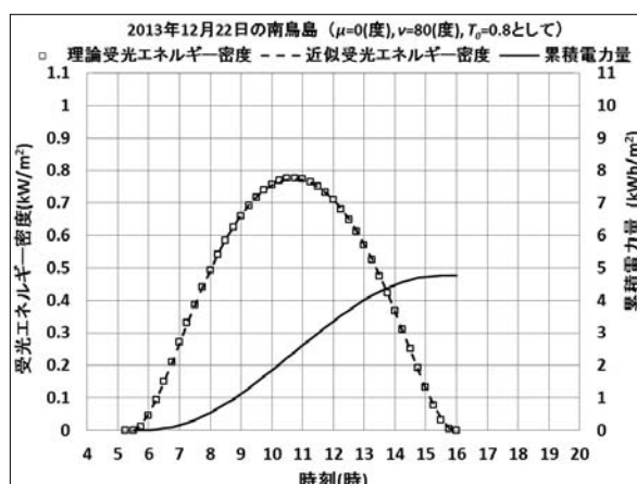
図20 2013年12月22日の南鳥島での受光エネルギー密度と累積電力量 ( \mu = 0 度、 \nu = 80 度、 T_0 = 0.8 )
