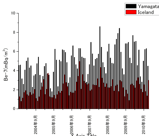
Fig1.2003 年からのアイスランドと山形の Be-7 濃度月変動の比較
