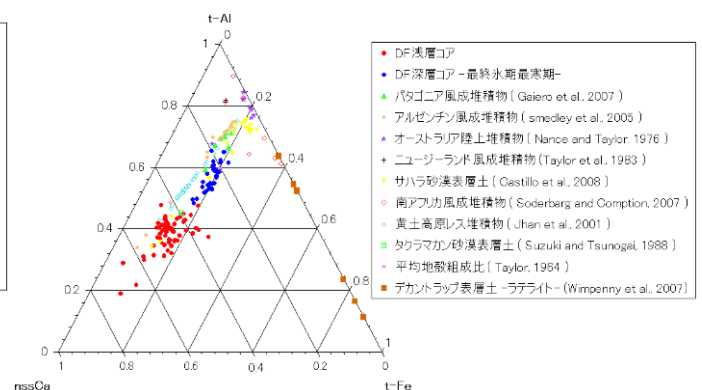
図2. 地殻表面物質およびDF氷コア中t-Al、t-Fe、nssCaの三角プロット
