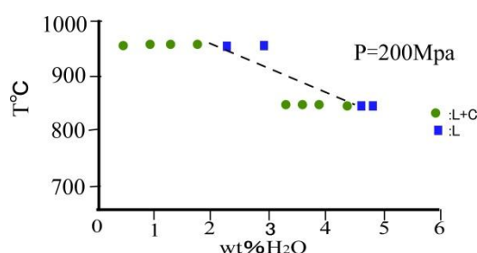
Fig.2. リキダス温度(200Mpa)
