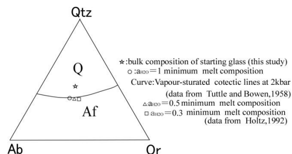
Fig.1. F Qtz-Ab-Or-H 2 O の相図(200Mpa)
