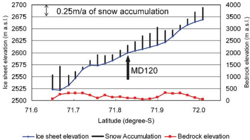
図6 GPS観測点MD120を中心にした氷床表面高度(青線)、岩盤高度(赤線)と、年間積雪収支量(縦棒)。データの間隔は約2km。矢印でMD120を示した。 Fig. 6. Ice sheet elevation, bedrock elevation and snow accumulation rate around MD120.
