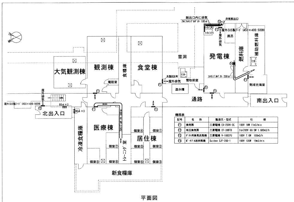
図 4 ドームふじ基地内の換気扇の仕様及び換気扇の通風方向（矢印で表記）
