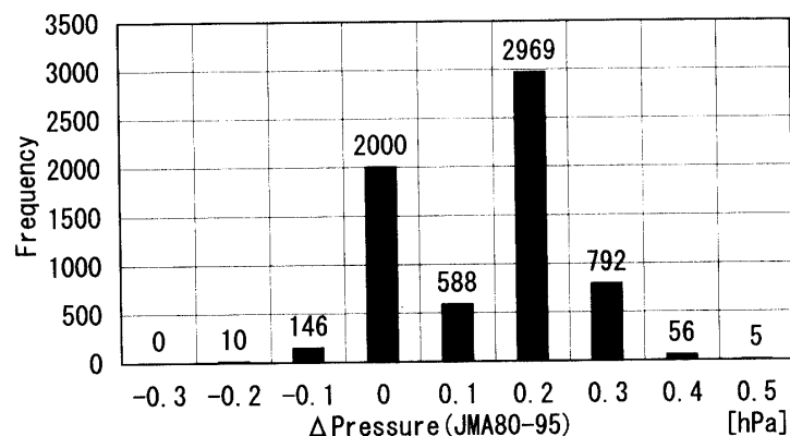
図4 気圧差のヒストグラム
