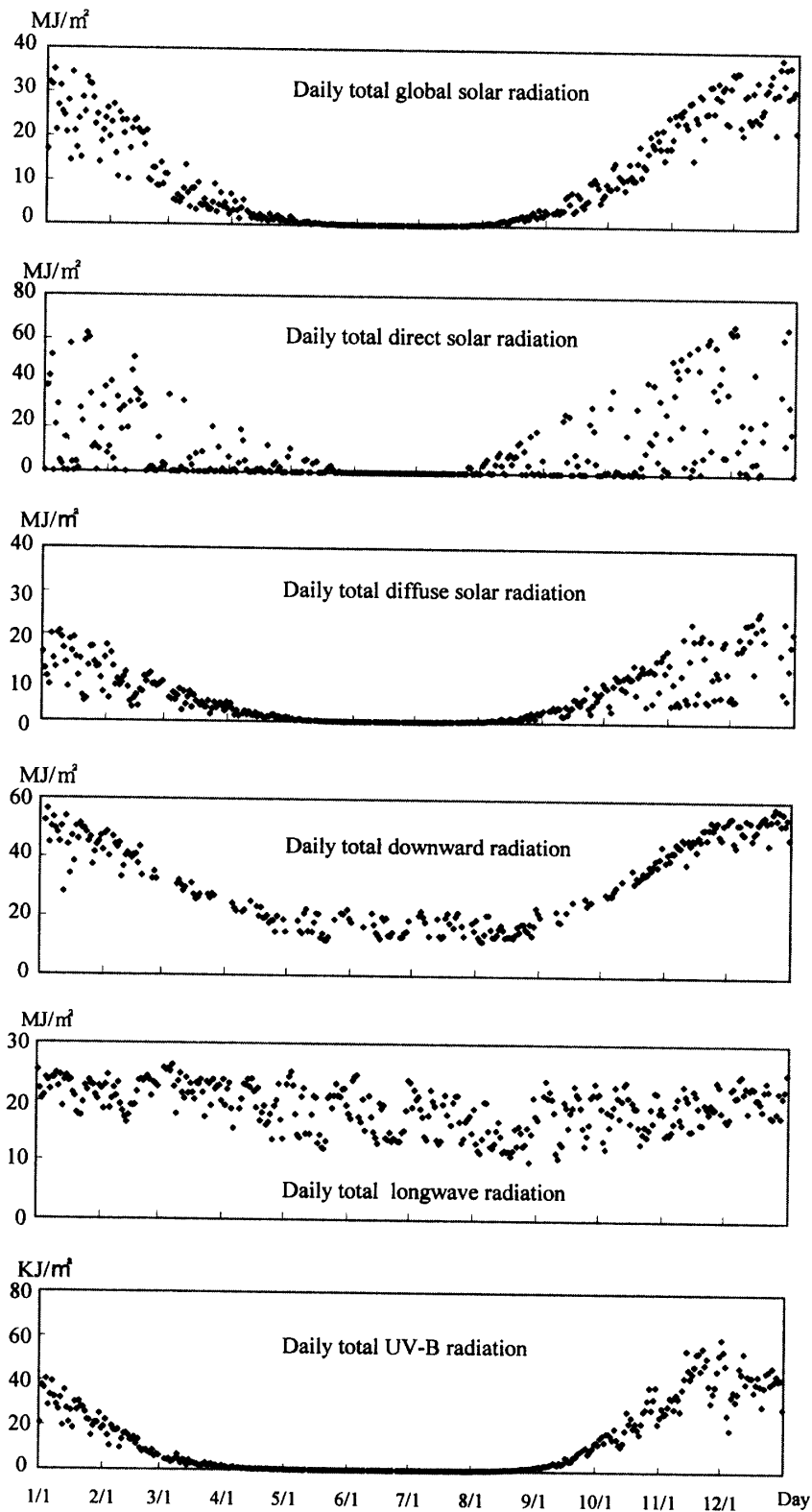
図 29 下向き放射観測結果 (1998 年)
