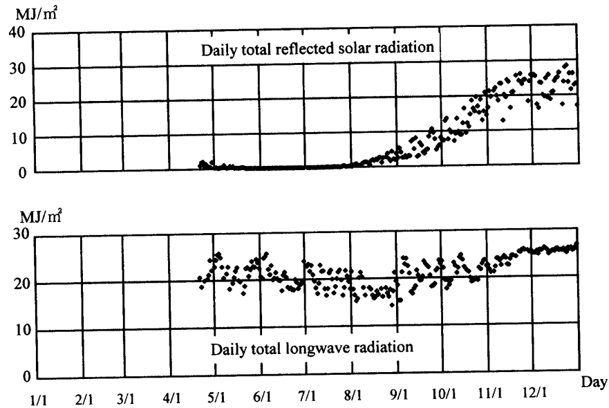
図 34 上向き放射観測結果 (1998 年) Fig. 34. Variations of upward radiation in 1998.
