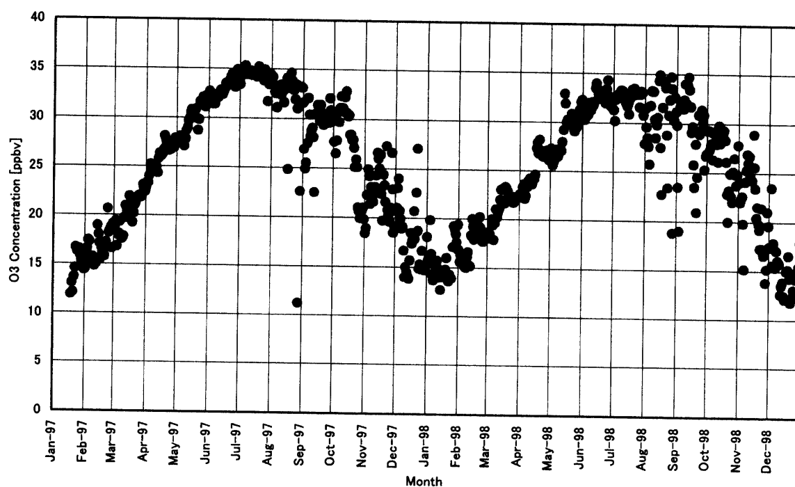
図 24 地上オゾン日別濃度値（1997-1998年）
