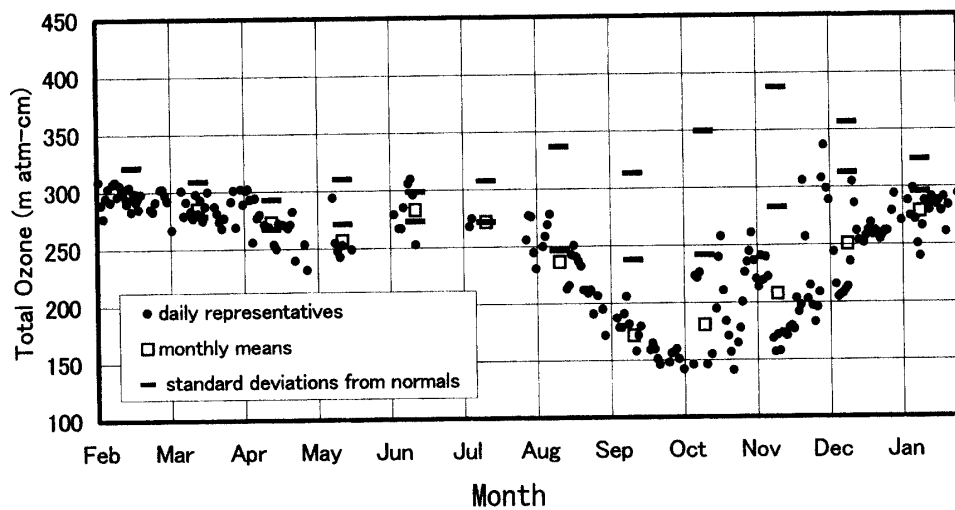
図 18 昭和基地におけるオゾン全量 (1998 年 2 月～1999 年 1 月) ●印は日代表値, □印は月平均値, — は平年値からの標準偏差 (上限・下限) をしめす。
