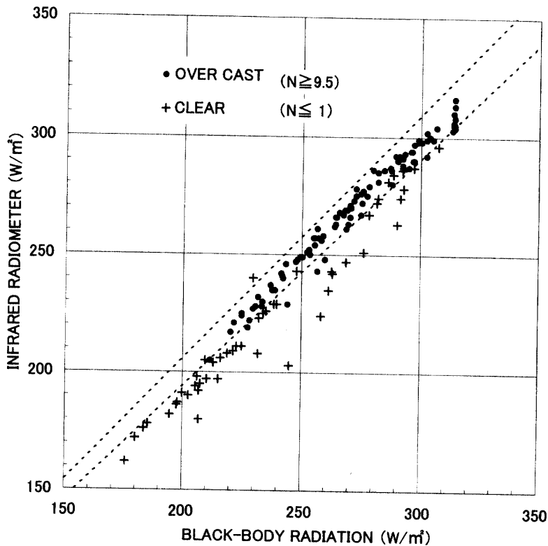
図 33 上向き長波放射量の比較 (赤外放射計による観測値と雪面温度を基に計算された黒体放射)
