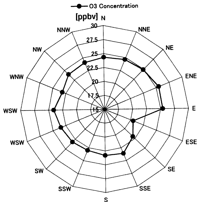
図 25 風向別地上オゾン濃度値（期間 1998 年 2 月 1 日～1999 年 1 月 19 日の 1 分値の平均値）
