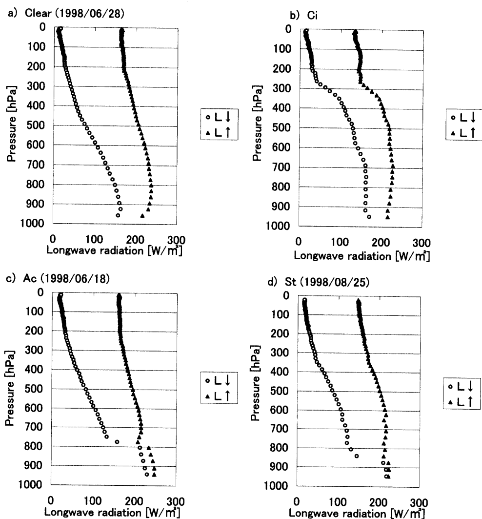
図 38 雲の種類による長波長放射鉛直プロファイルの比較 a) は快晴 (雲量 0), b) は上層雲で覆われた場合 (Ci), c) は中層雲で覆われた場合 (Ac), d) は下層雲で覆われた場合 (St).
