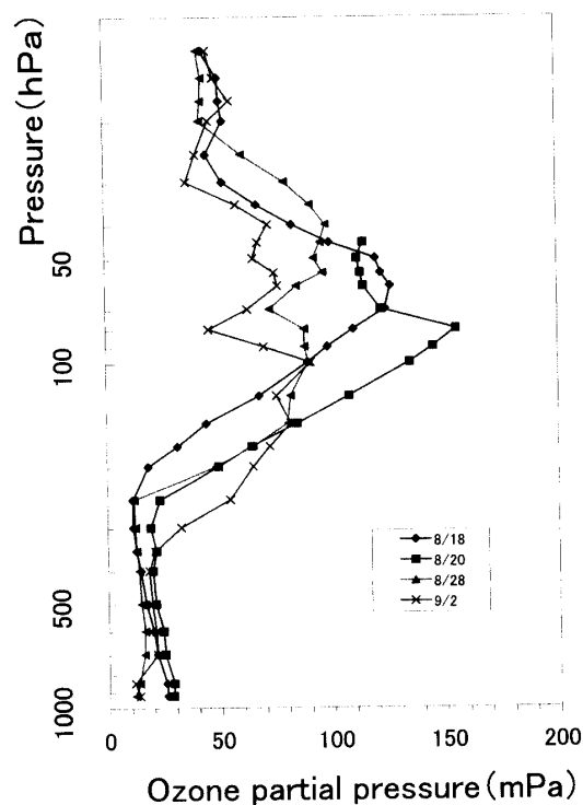
図27 地上オゾン濃度急減現象発生前後のオゾンゾンデ観測値 Fig. 27. Ozonesonde data during the low ozone episode.
