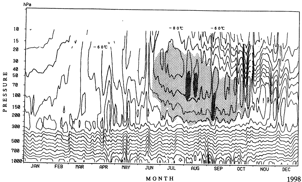
図 39 昭和基地における気温の時間高度断面図（1998 年）影の部分は NAT が析出する（硝酸 10 ppbv, 水蒸気 5 ppmv を仮定）温度域, 濃い影の部分は氷（水蒸気 5 ppmv を仮定）が析出する温度域
