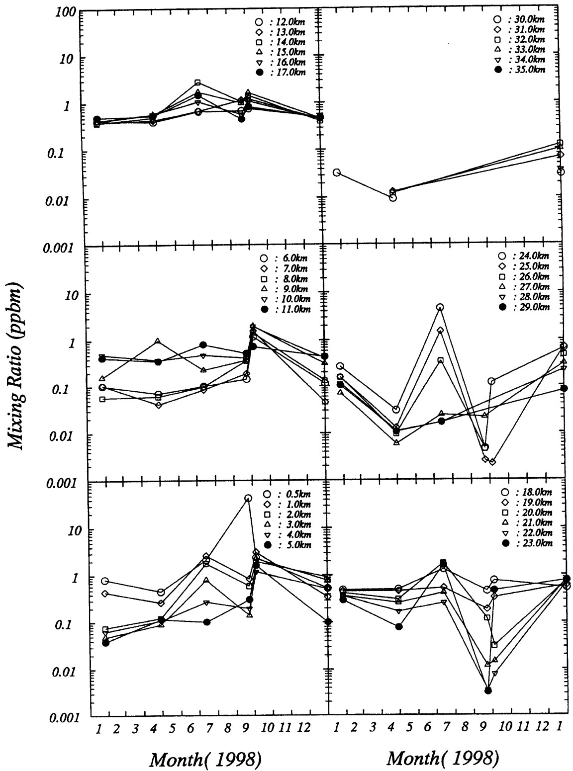
図 40 重量混合比の時間変化
