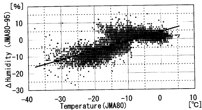
図7 相対湿度差と80型気温の関係
