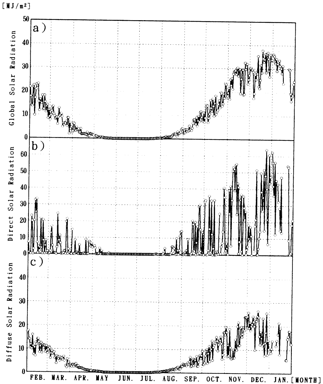
図 14 日射量日積算値の年変化 (1993 年 2 月-1994 年 1 月)
