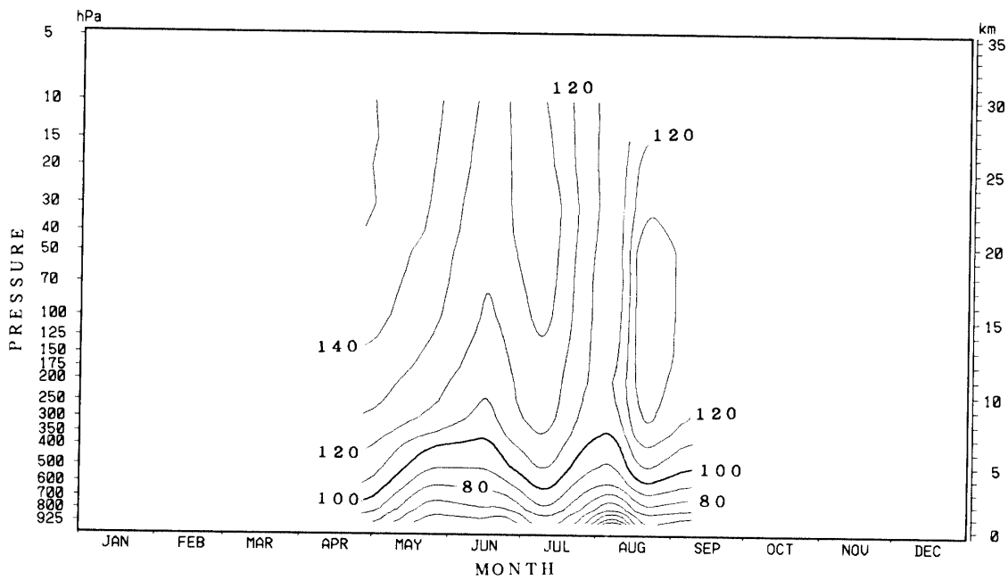
図 24 輻射ゾンデによる正味放射量の変化 Fig. 24. Variations of net flux of infrared radiation ( W/m^2 ) by radiometersonde in 1993.
