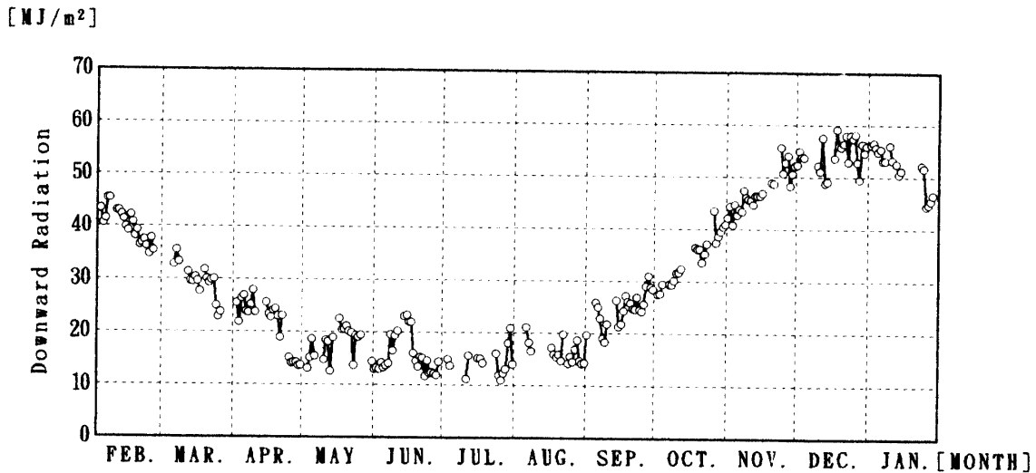
図 16 下向き放射量日積算値の年変化 (1993 年 2 月-1994 年 1 月)
