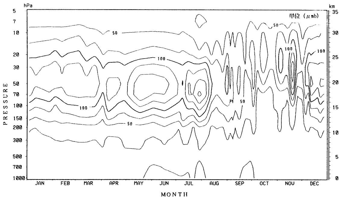
図 9 オゾン分圧の鉛直分布の年変化 (気象庁オゾン層解析室作成)
