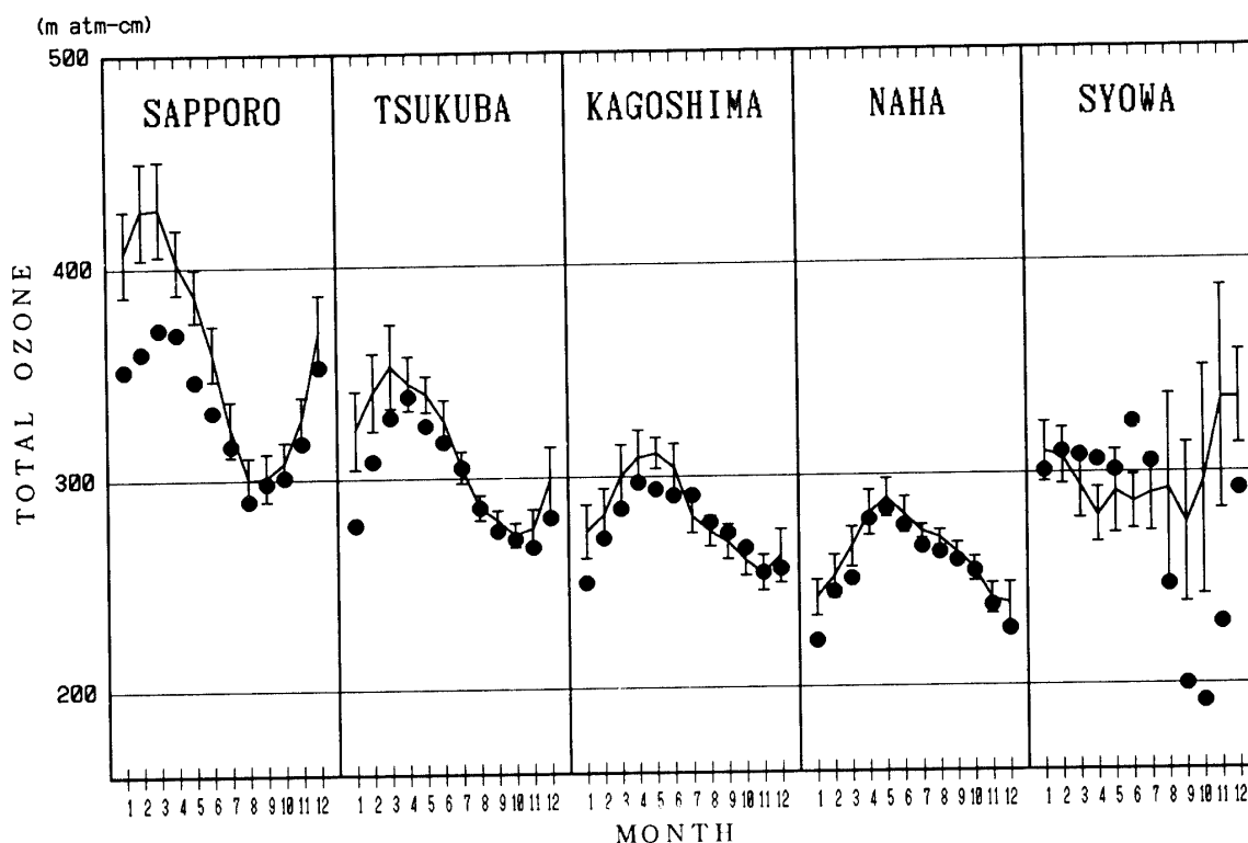
図7 オゾン全量月平均値（1993年）と月別累年平均値（1961-1990年）（気象庁オゾン層解析室作成）
