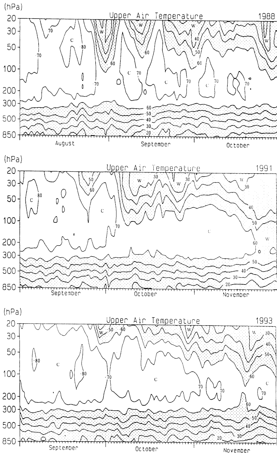
図 4 上層気温の変化 (1988 年 8 月-10 月, 1991 年 9 月-11 月, 1993 年 9 月-11 月) Fig. 4. Variation of upper air temperature in °C (August–October 1988, September–November 1991, September–November 1993).
