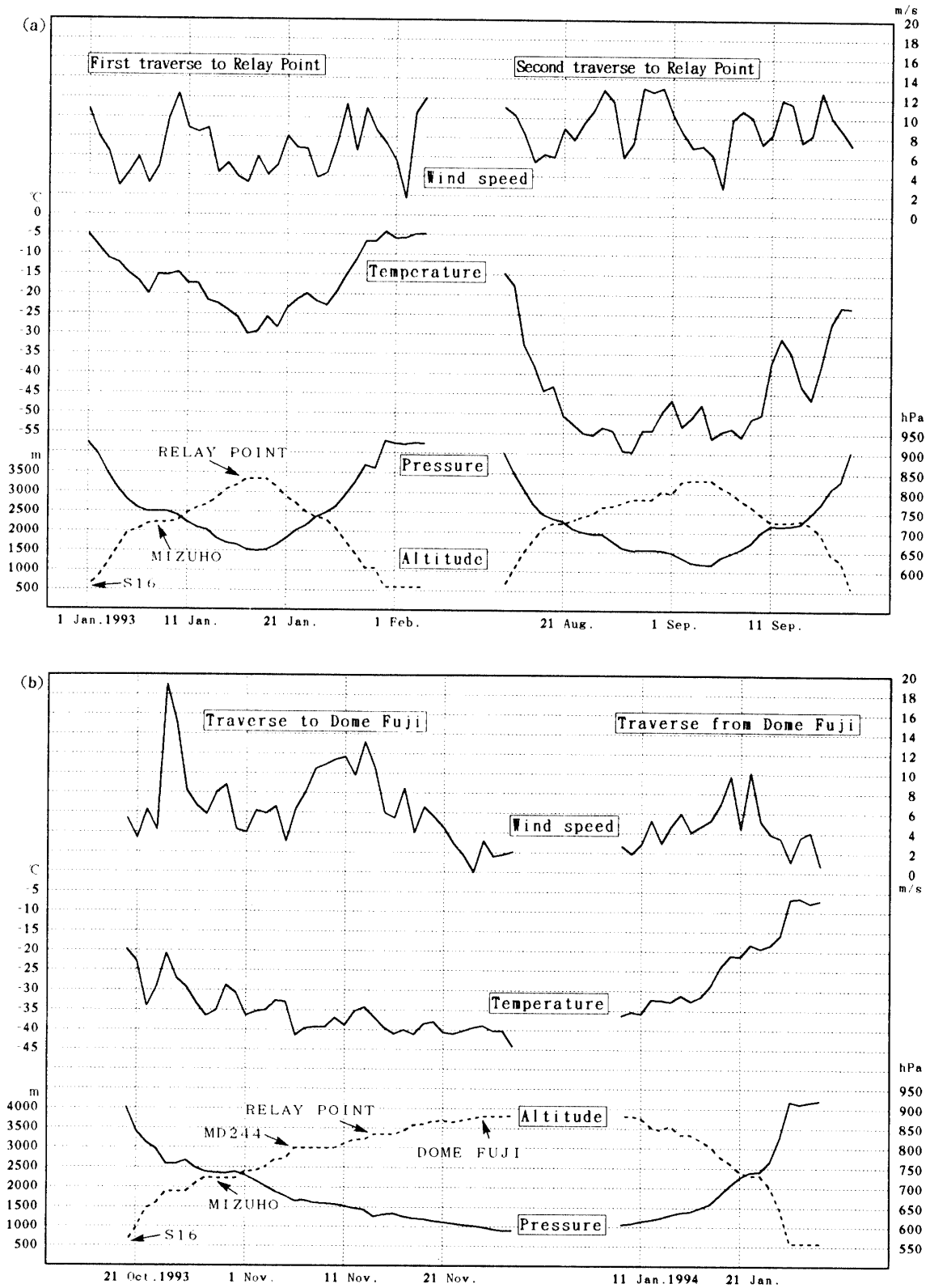
図 29a, b. 中継拠点旅行中 (a) とドームふじ観測拠点旅行往復路 (b) の標高と気象データの経過 (21 LT) Fig. 29a, b. Altitude and surface meteorological data during two traverses to Relay Point (a) and traverse to Dome Fuji Station (b).
