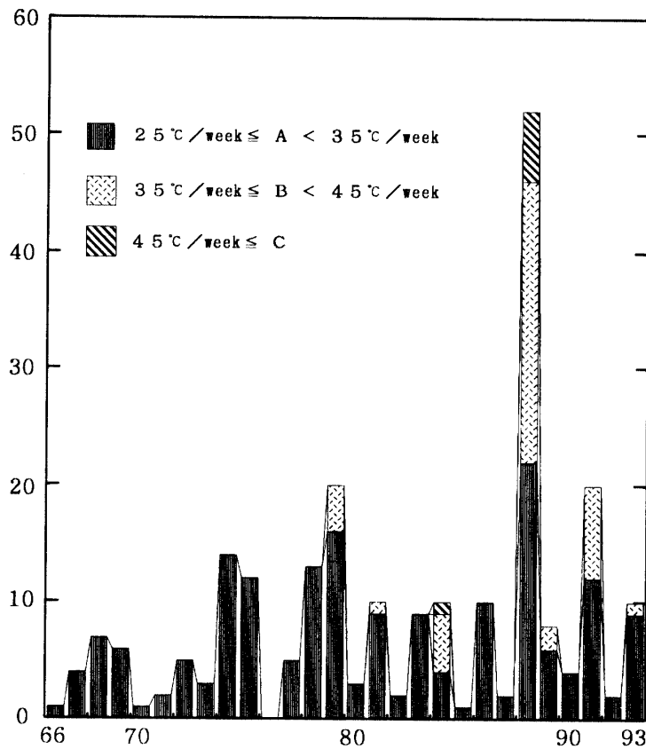
図 6 指定気圧面における成層圏突然昇温統計結果 (1966 年-1993 年)
