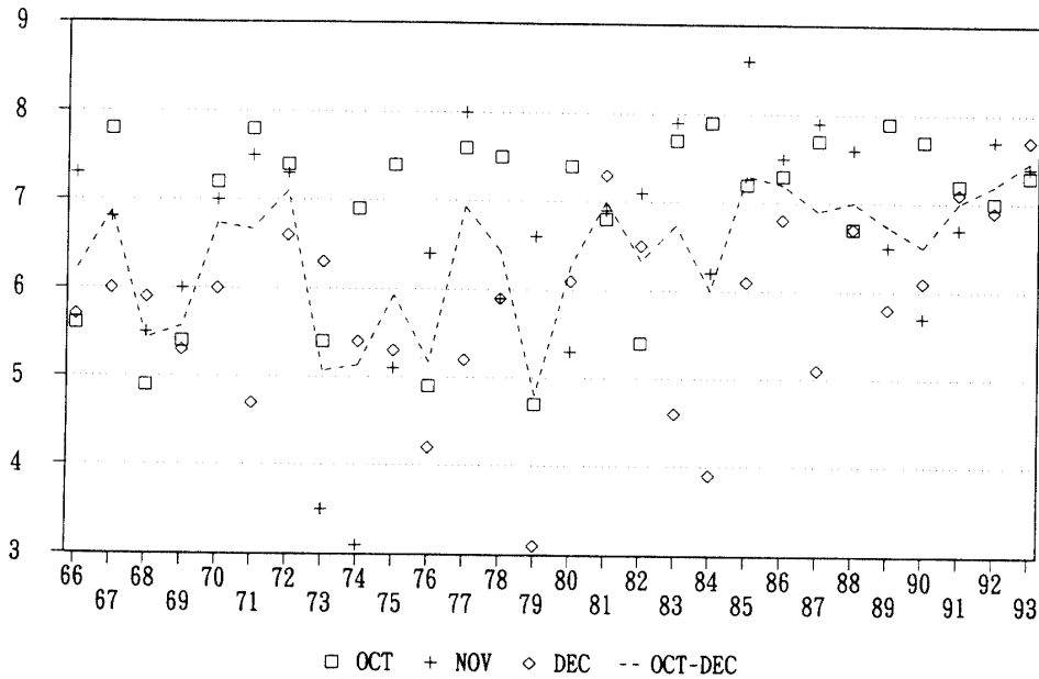
図 26 10-12月雲量の経年変化
