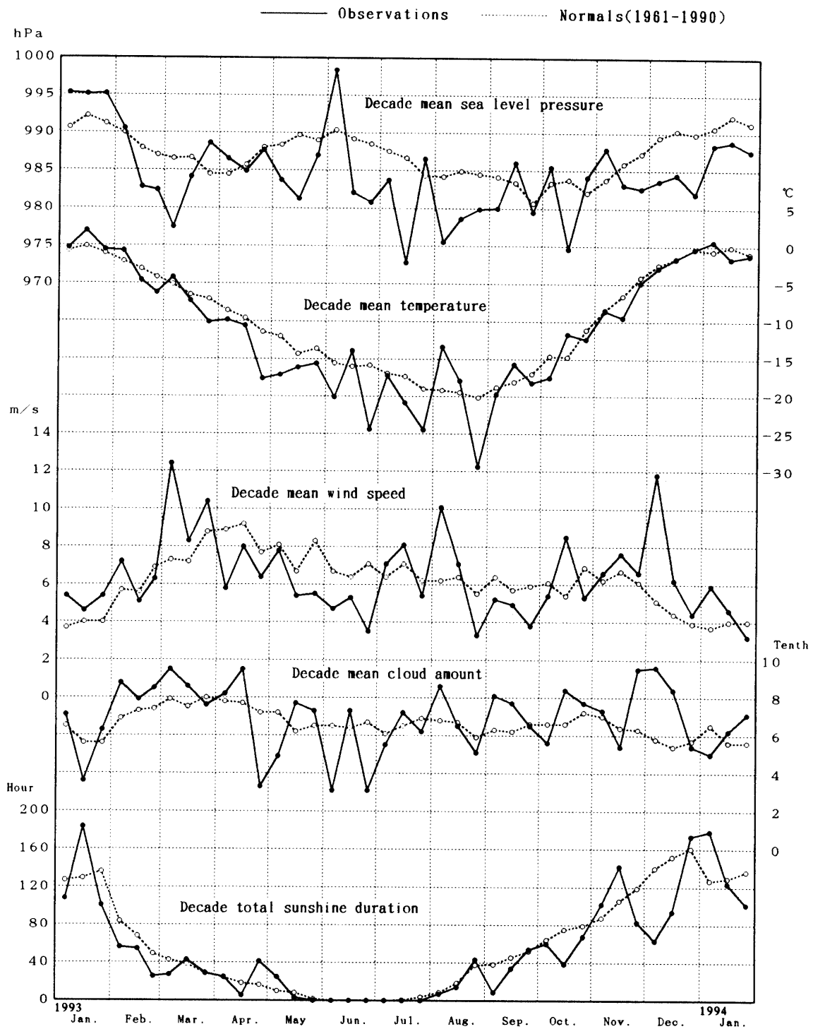
図 1 地上気象旬別値年変化 (1993 年 1 月-1994 年 1 月)
