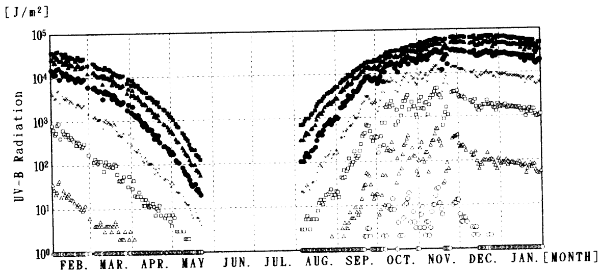
図 21 5 nm 帯別平均 UV-B 日積算値の年変化 (1993 年 2 月-1994 年 1 月)
