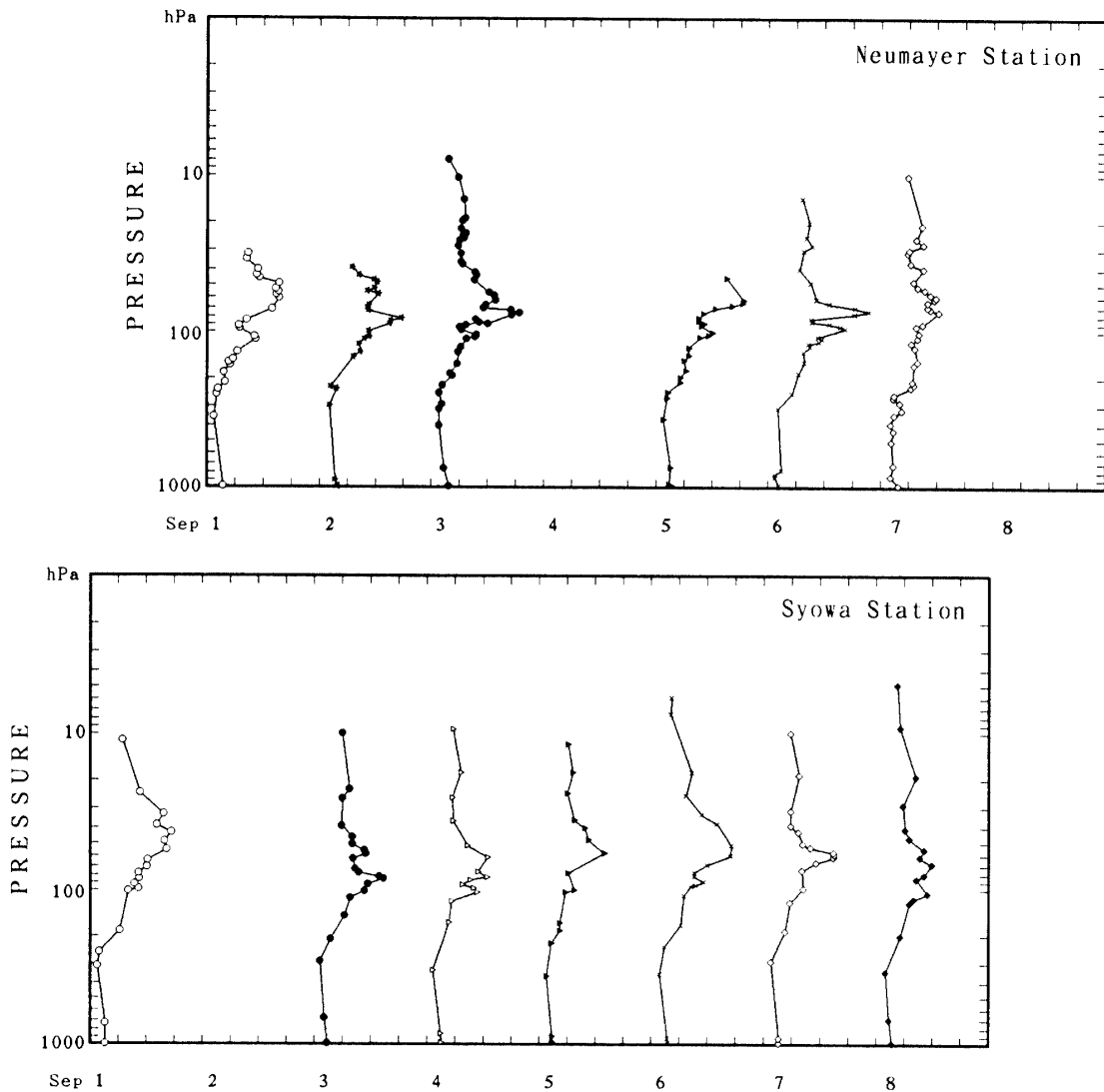
図 12 ROSA93 期間中のオゾン分圧の高度分布 (1993 年 9 月 1-8 日)
