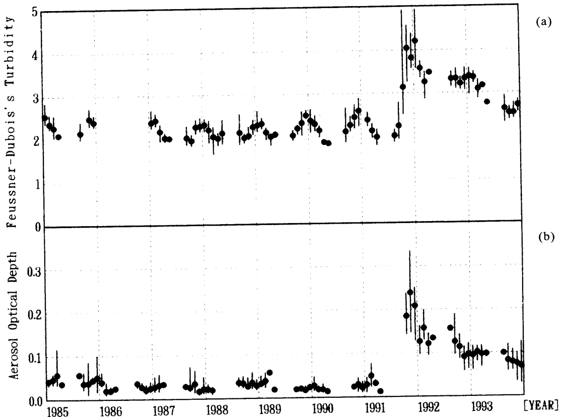
図 23 大気混濁度の経年変化 (1985-1993 年)
