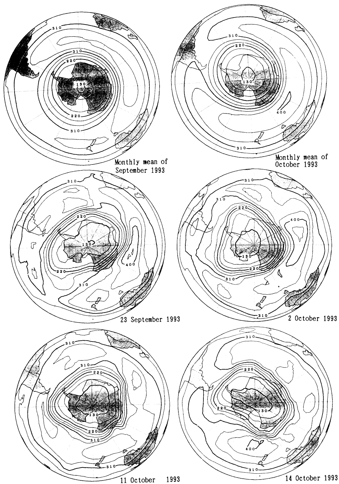
図 13 TOMS による 1993 年の南半球オゾン全量分布図 (気象庁オゾン層解析室作成) Fig. 13. Maps of total ozone in the Southern Hemisphere by TOMS.
