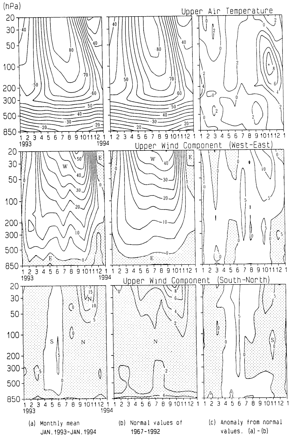
図3 月平均気温と高層風の東西成分・南北成分の年変化。(a) 1993年平均, (b) 累年平均および(c) 累年平均からの偏差
