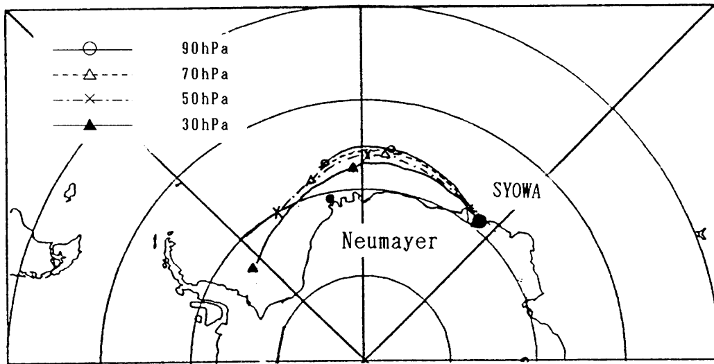
図 11 昭和基地上空に到達した気塊の流跡線 (1993年9月3日12 UT から12時間前および24時間前)
