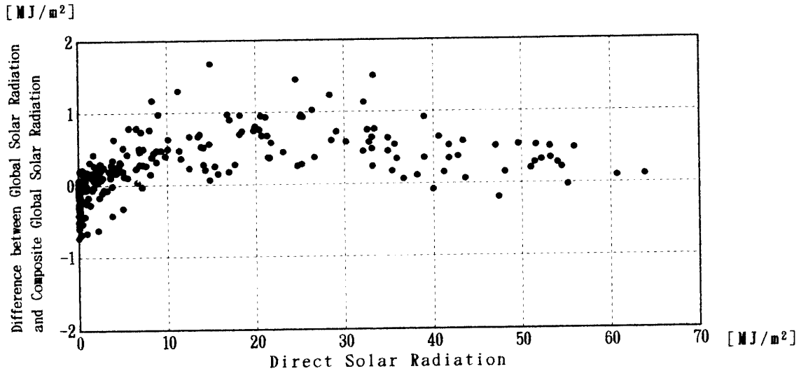
図 15 直達日射量と全天日射量観測精度（全天日射量-合成全天日射量）の関係（1993年2月-1994年1月）
