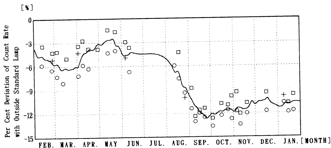
図 18 外部標準ランプ計数率偏差の年変化と感度トレンド (1993 年 2 月-1994 年 1 月)
