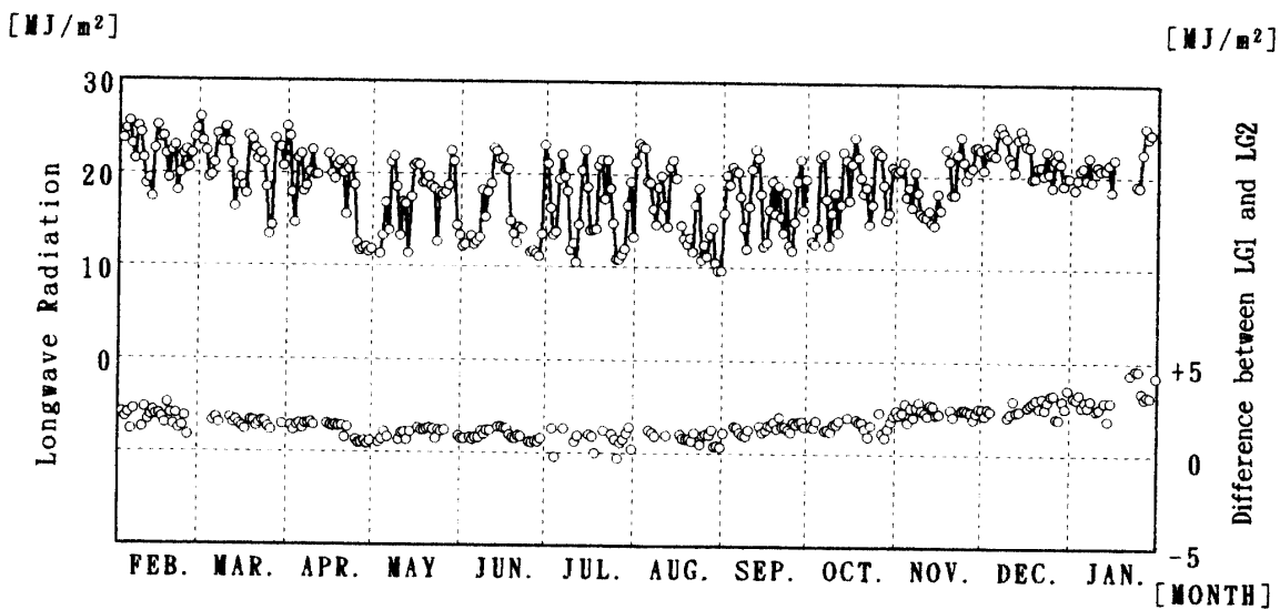
図 17 長波長放射量日積算値 (LG1) と長波長放射量精度 (LG1-LG2) の年変化 (1993 年 2 月-1994 年 1 月)
