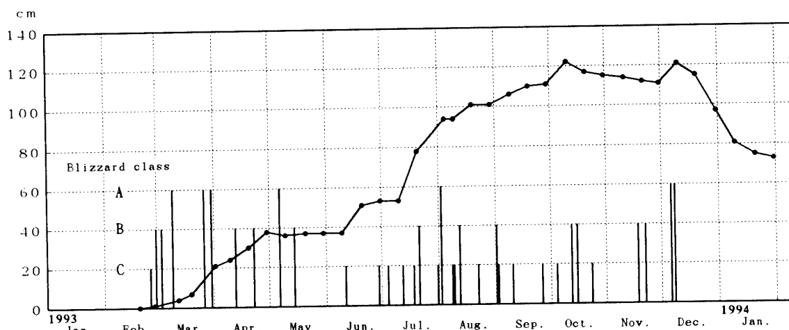
図 2 積雪量の年変化とブリザード (1993 年 2 月-1994 年 1 月)
