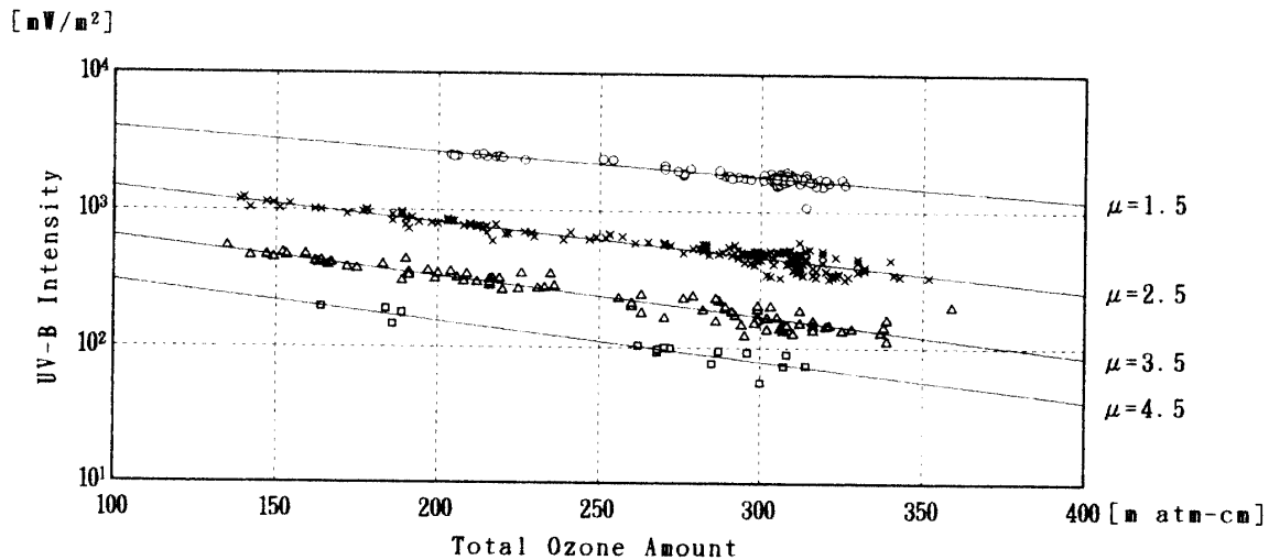
図 22 オゾン全量と UV-B 強度の関係 (1993 年 2 月-1994 年 1 月)
