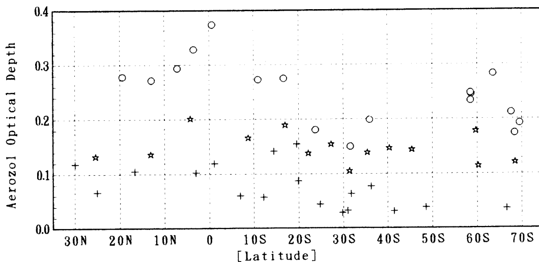
図 31 船上におけるサンフォトメーターによるエアロゾルの光学的厚さ (500nm) の緯度分布 Fig. 31. Latitude distribution of aerosol optical depth at 500nm observed on board with sunphotometer. +, O, ☆ show the data of 1979-1981, 1991, 1992 respectively.
