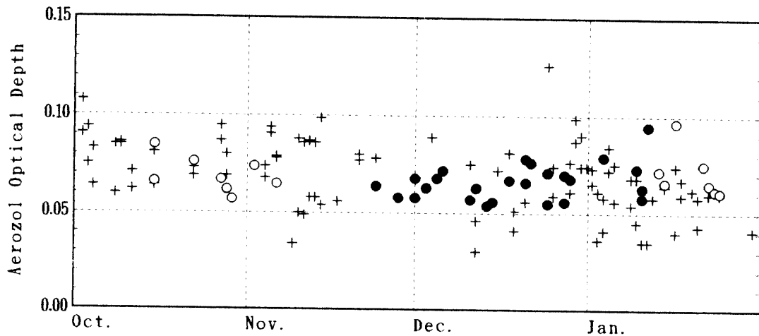
図 32 内陸と昭和基地におけるサンフォトメーターによるエアロゾルの光学的厚さ (500 nm) の時系列 (1993 年 10 月-1994 年 1 月)
