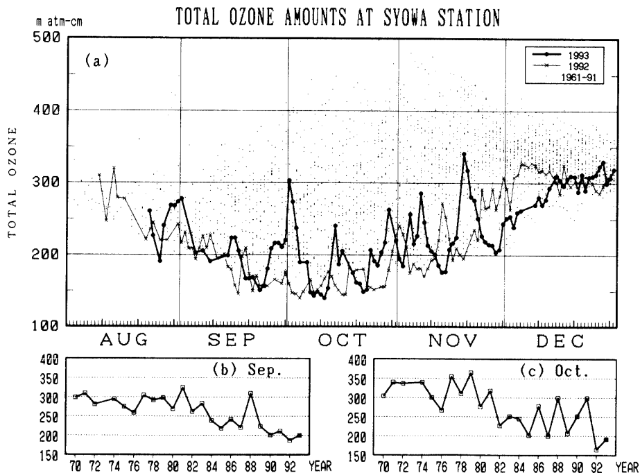
図 8 オゾン全量日別値 (a) および 9 月、10 月の月平均値の経年変化 (b, c) (気象庁オゾン層解析室作成)
