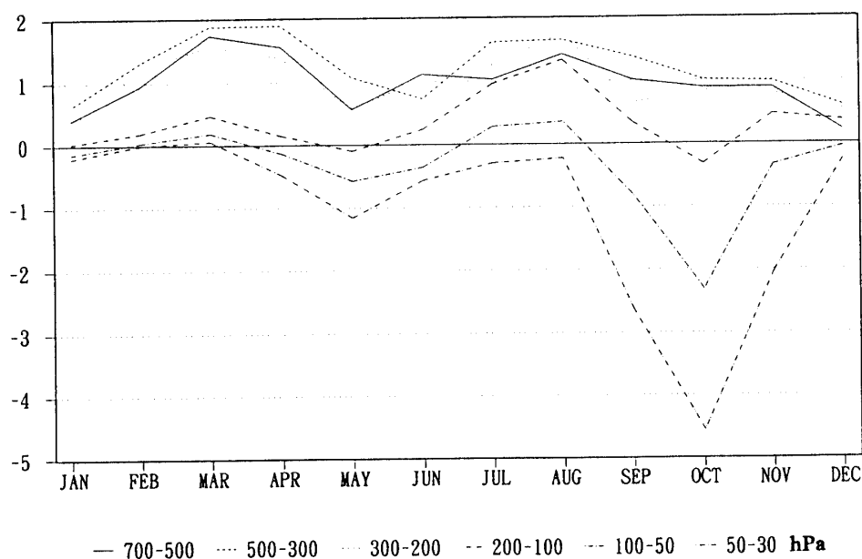
図 27 昭和基地上空への温度移流量年変化 月平均値の累年平均値 (1967 年–1993 年). 単位は ^\circ\text{C}/\text{日}
