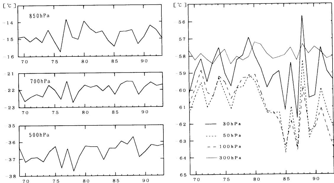
図5 年平均指定気圧面気温の経年変化(1969年–1993年)
