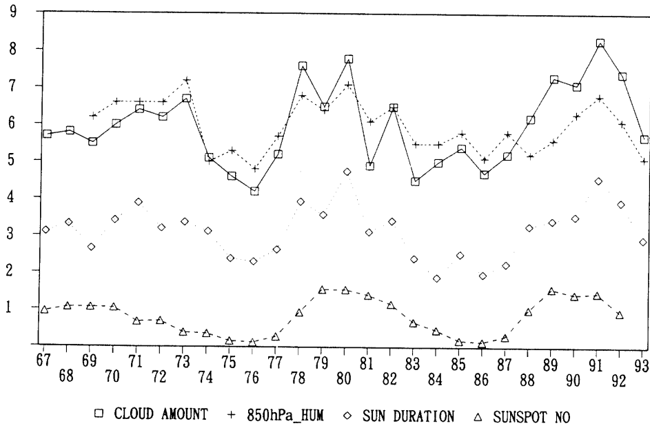
図 25 1月の月平均気象量と年平均黒点数の経年変化
