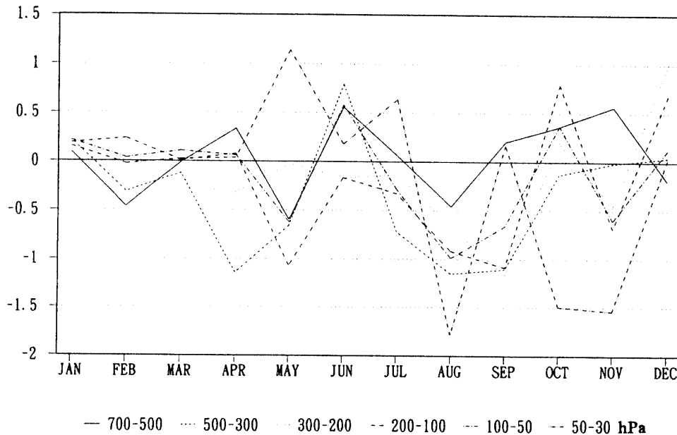
図 28 昭和基地上空への温度移流量年変化
