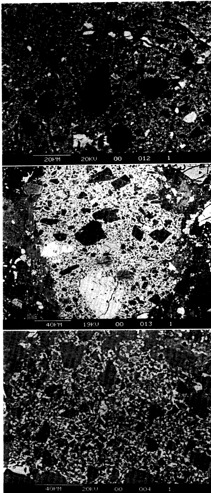
Fig. 4. Crystalline impact melt breccias: plagioclase (dark gray), olivine and pyroxene (light gray).
