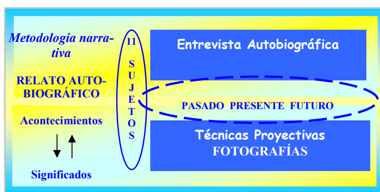
Figura 1. Retícula contenedora
