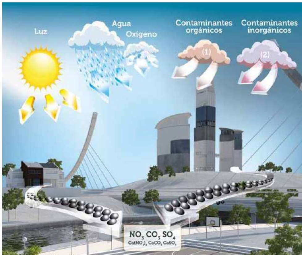
Fig. 6 “Esquema del proceso de oxidación de los cementos fotocatalíticos” Fuente: FYM-Italcementi Group.
