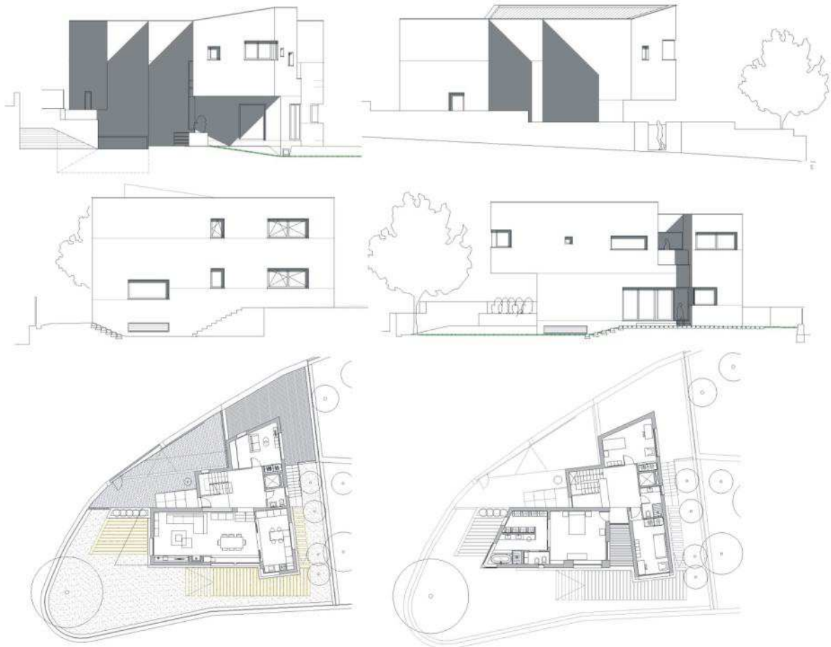
Fig. 3 “Fachadas y plantas de la vivienda” Fuente: Autor.
