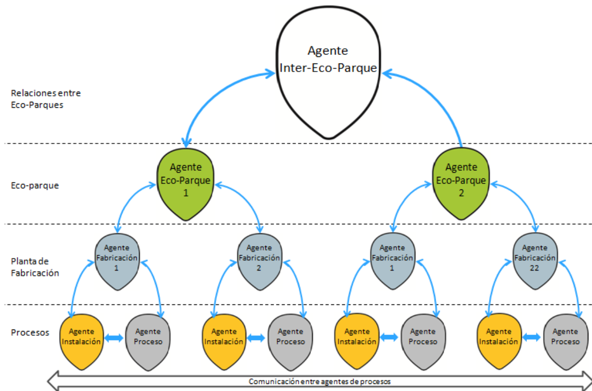
Figura 5. Estructura de comunicación entre agentes
