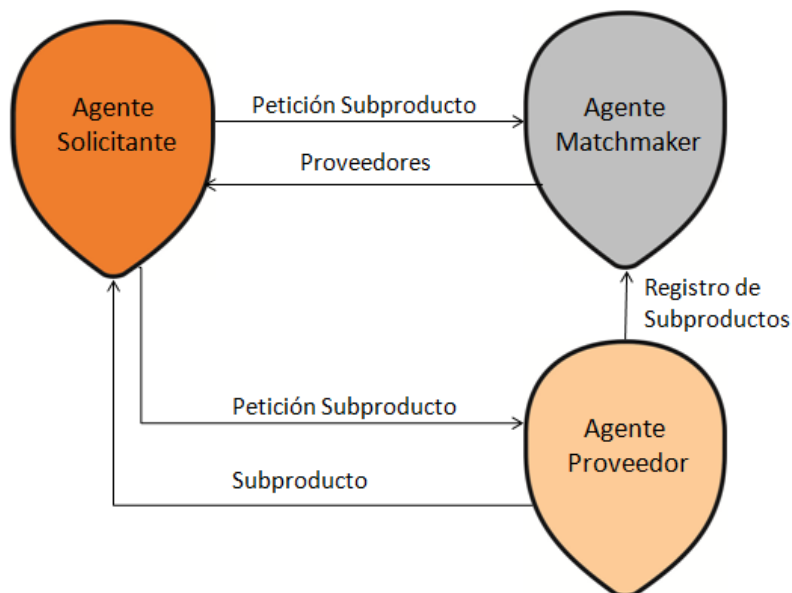
Figura 3. Arquitectura de sistema multiagente por Matchmaker
