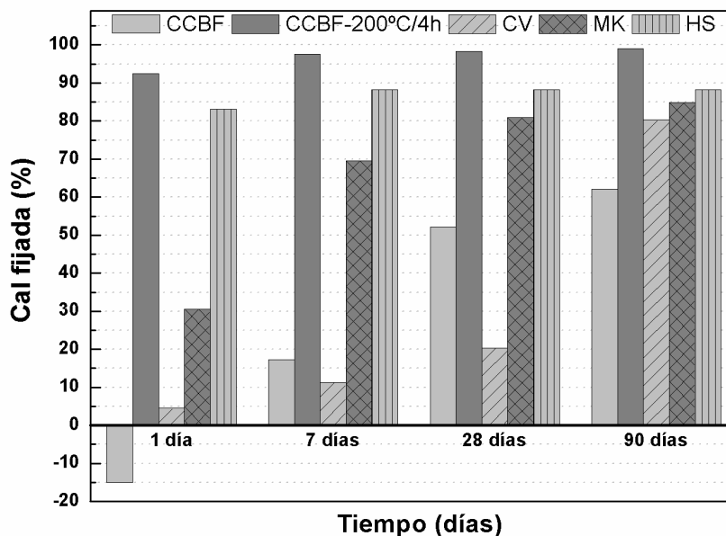
Figura 2. % Cal fijada de la ceniza CCBF y la ceniza CCBF-200 ^\circ\text{C}/4\text{h} en medio NaOH 1M a diferentes tiempos de reacción.
