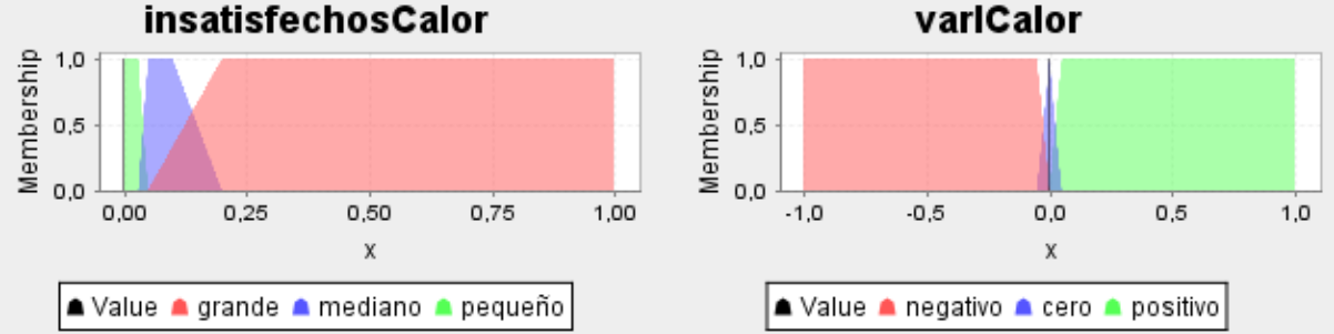
Figura 2. Funciones de pertenencia cuando no hay confort por calor y la variación éste.
