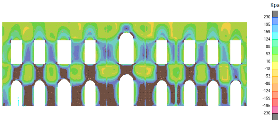
Figura 12: Envoltura de las tensiones de corte en fachada Norte producto de análisis Tiempo Historia
