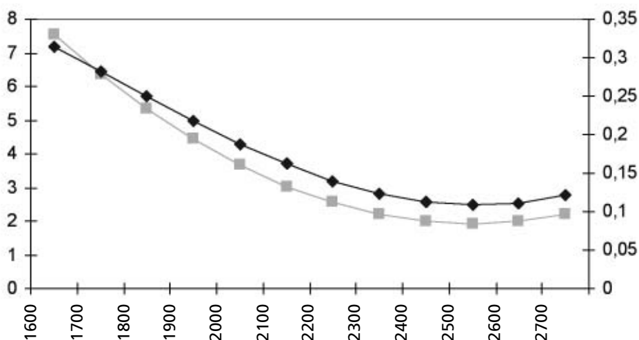
Figura 1. Representación de la varianza genética ( \square ) y la heredabilidad ( \diamond ) según la distancia utilizando la media kilométrica en Trotador Español.
