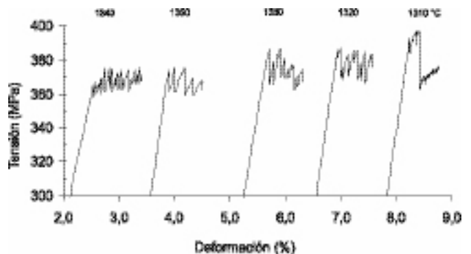
Fig. 1.- Curva tensión-deformación con inestabilidades plásticas de una muestra con 24 mol% Y 2 O 3 , a velocidad de travesa de 5\cdot 10^{-4} \text{m}\cdot\text{s}^{-1} . Se muestran distintos tramos con temperaturas entre 1310 y 1350°C.
