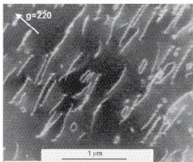
Fig. 3.- Micrografía de MET del plano primario (001) de una muestra con 24 mol% \text{Y}_2\text{O}_3 con un 3% de deformación, mostrando subestructura de dislocaciones.
