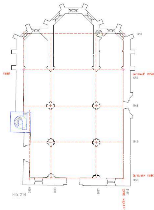
Fig. 4. Estudio del trazado de Santiago
