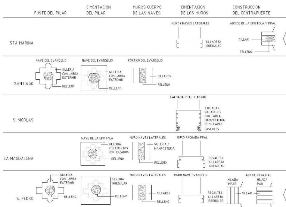
Fig. 6. Soluciones constructivas de distintos edificios: pilares, muros, contrafuertes y sus cimentaciones
