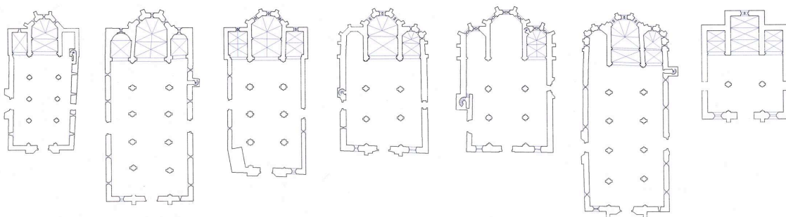
Fig. 1. Planta de las iglesias parroquiales de Córdoba (restitución omitiendo añadidos al edificio medieval)
