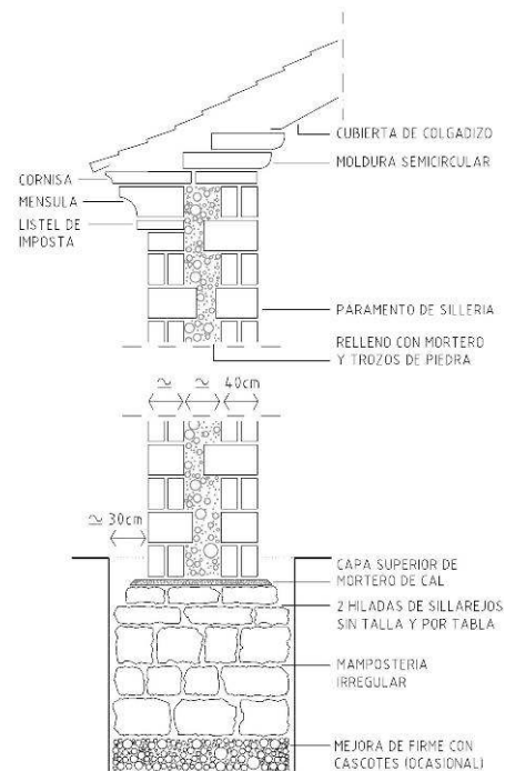
Fig. 8. Sección constructiva “tipo” de muro de fachada
