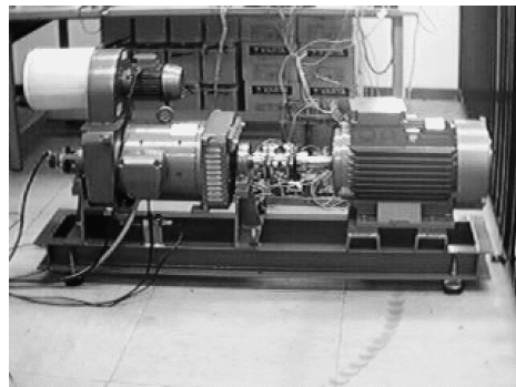
Figure 9. Ac-motor test-rig.
