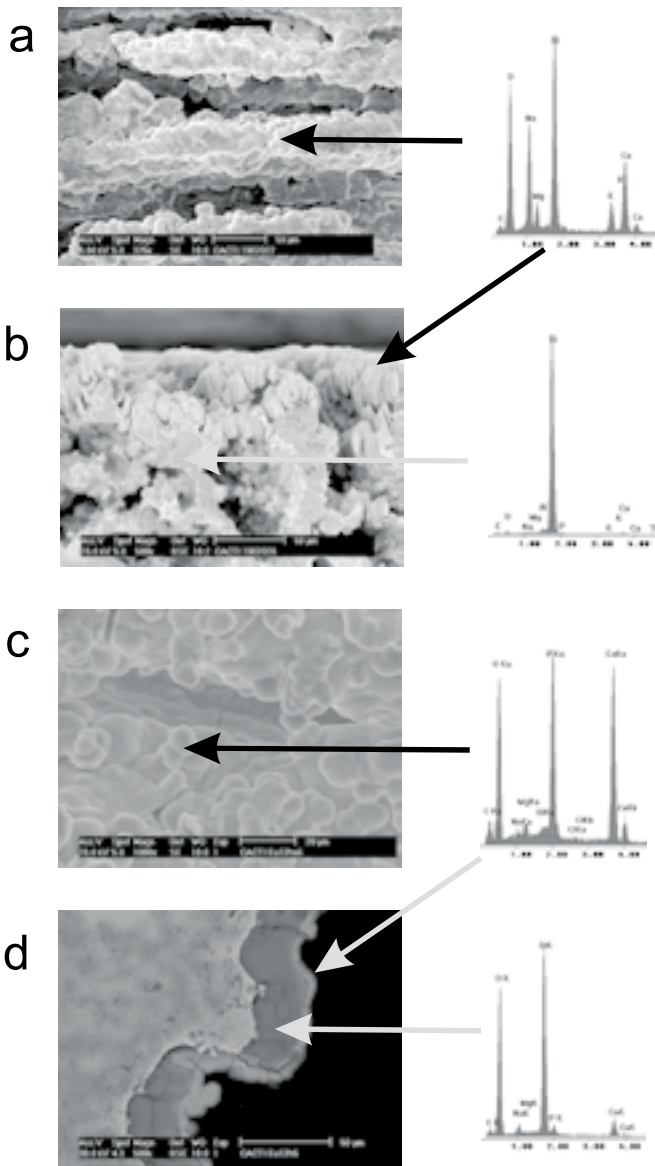
Fig. 2- Micrográficas SEM y análisis EDS de las capas de vidrio bioactivo producidas por PLD sobre SiC biomórfico, (a) vista de la superficie, y, (b) sección. (c) y (d) muestran una vista de la superficie y la sección, respectivamente, de los cambios originados en la capa de vidrio tras la inmersión en SBF durante 72 h.
