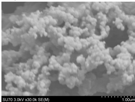
NPOF-1
