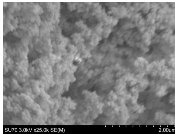
NPOF-1-NO 2
