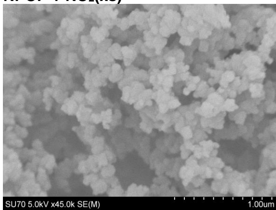
NPOF-1-NH 2 (xs)
