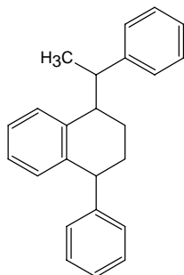
Styrene Trimer
