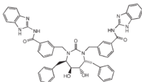
SD146 (1QBT)
