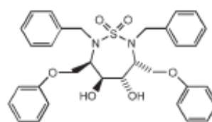
Aha006 (1AJV)
