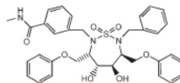
Aha047 (1G2K)
