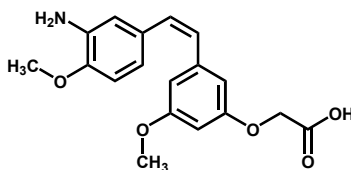
VT54
