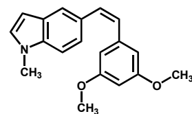
GG 251
