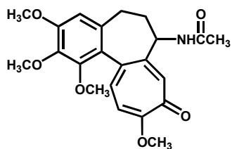
Colchicine
