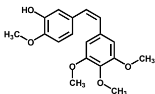
Combretastatin
