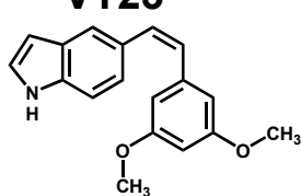
GG 247
