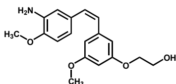
VT23
