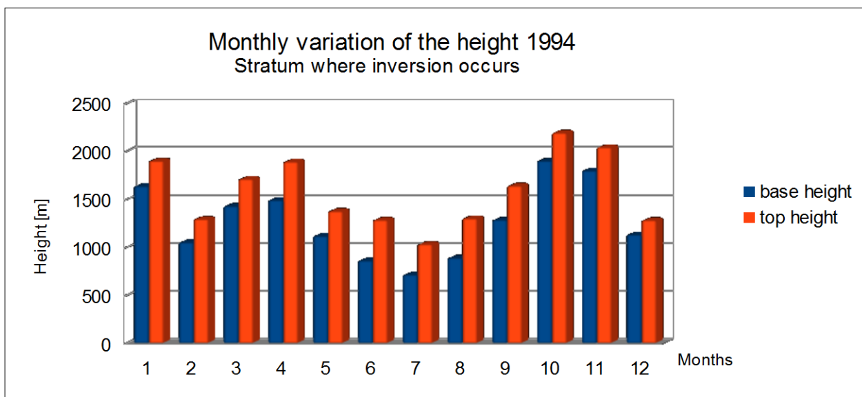
Gráfico 5. Variación mensual de la altura de la capa de inversión térmica para 1994, 1.
