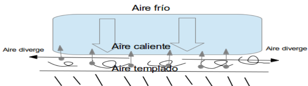
Figura 14. Esquema inversión térmica de subsidencia en los meses fríos y calurosos.
