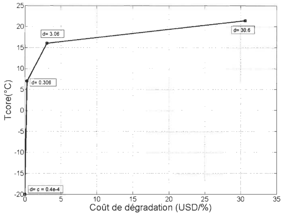
Figure 4. 8 Graphique de la température limite en fonction de la dégradation des coûts.
