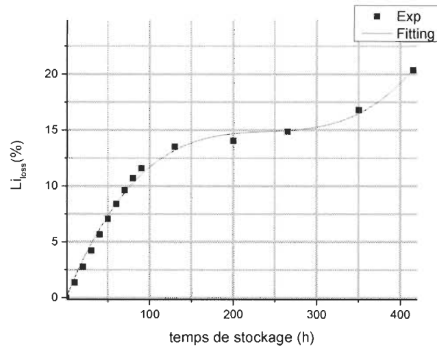
Figure 3.15 Modélisation des pertes calendaires par « fitting » polynomial.
