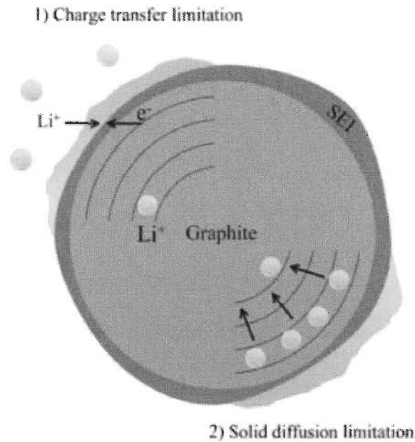
Figure 3. 12 Principe du modèle de vieillissement de Legrand [145].
