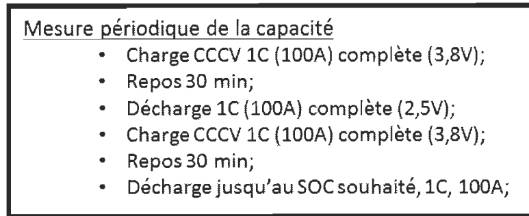
Figure 3. 2 Protocole pour la caractérisation périodique.
