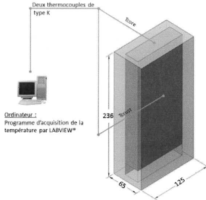
Figure A.2 Emplacement des différents thermocouples sur la cellule \text{LiFeMnPO}_4 avec T_{core} : température d'une électrode et T_{crust} température de la surface.
