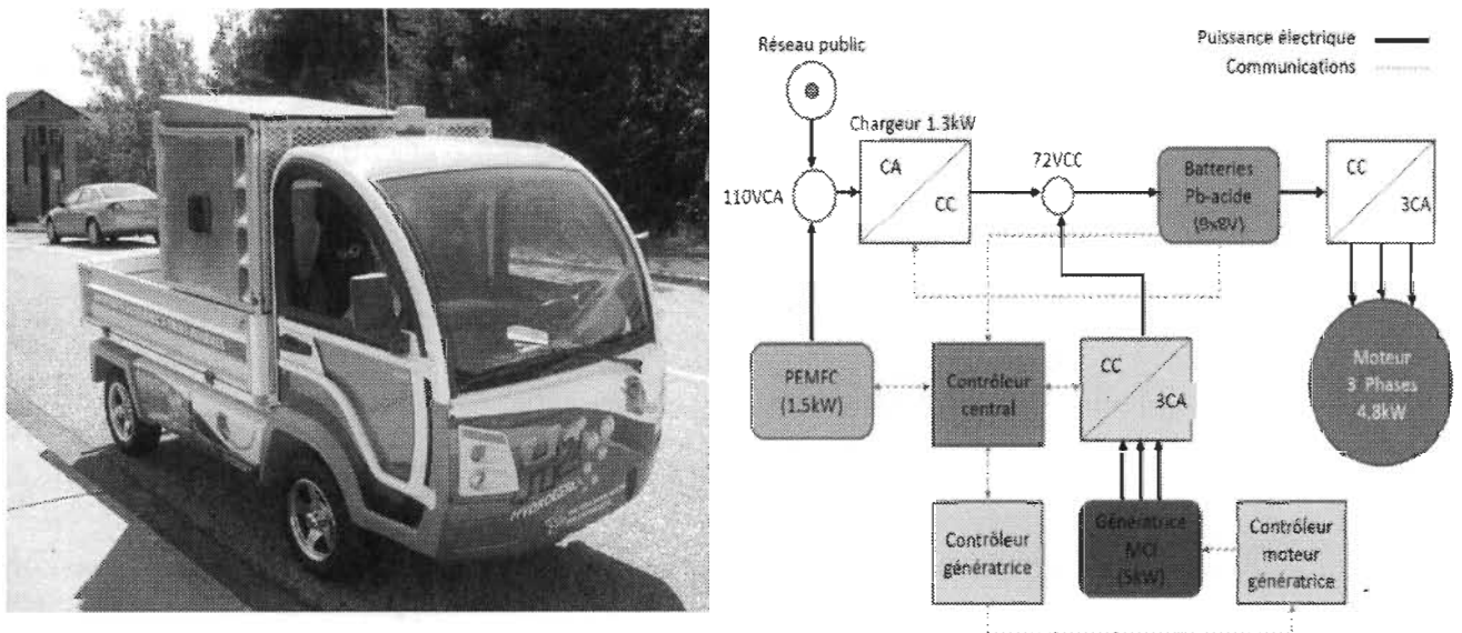
Figure B. 1 À gauche, VEH NÉMO modifié. A droite, architecture du NÉMO modifié.
