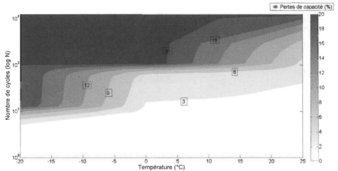
Figure 3. 16 Modélisation des pertes par cyclage. Le modèle n'est plus valide au-delà du critère de fin de vie (pertes de capacité supérieures à 20%).
