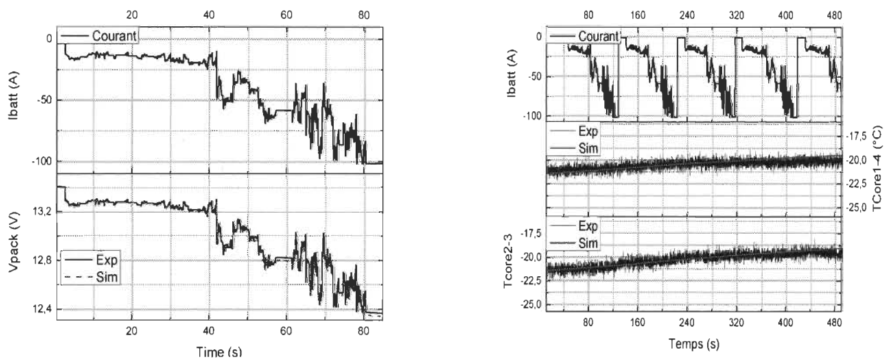
Figure 2. 28 Deuxième validation du modèle. À gauche : courbes expérimentale et de simulation de la tension de la cellule sous un courant aléatoire à 0°C. A droite : courbes expérimentale et de simulation de la température de la cellule sous un courant aléatoire à -20°C.
