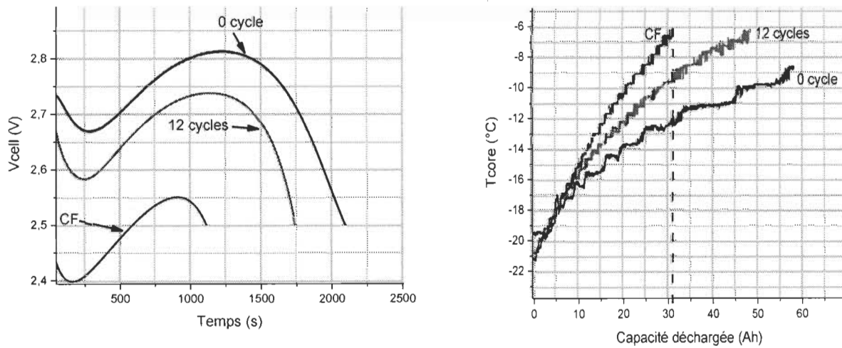
Figure 3.5 Résultat du vieillissement par cyclage à -20°C. À gauche : évolution des capacités. À droite : évolution de la température.
