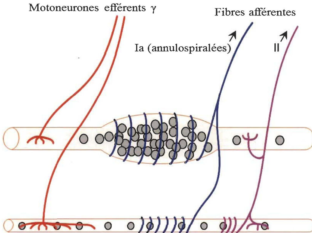
Figure 1. Fuseau neuromusculaire
