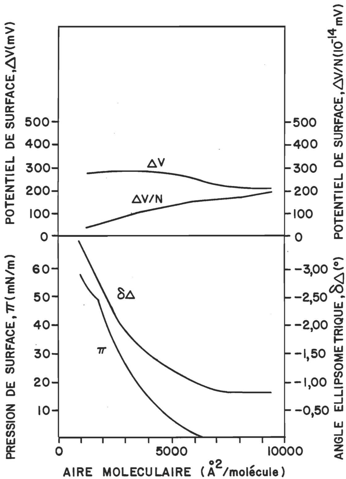
Figure 24. L'isotherme de pression, de potentiel de surface et ellipsométrique de la rhodopsine intacte à l'interface azote-eau. La température est maintenue à 17,0 \pm 0,5^\circ\text{C} .
