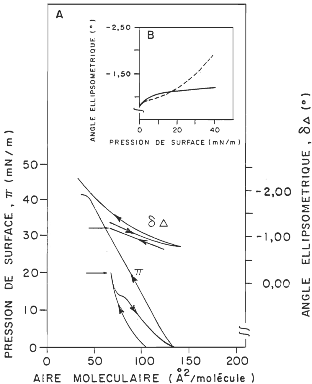
Figure 31. A: L'isotherme de pression de surface et ellipsométrie de la PC des SEB en absence (compression) et en présence de G-protéine (décompression et recompression) à l'interface azote-eau. La température est maintenue à 19,0 \pm 0,5^\circ\text{C} . B: Le graphique de l'angle ellipsométrique en fonction de la pression de surface pour la PC des SEB (—) et pour la recompression du film de PC des SEB-G-protéine (- - -).
