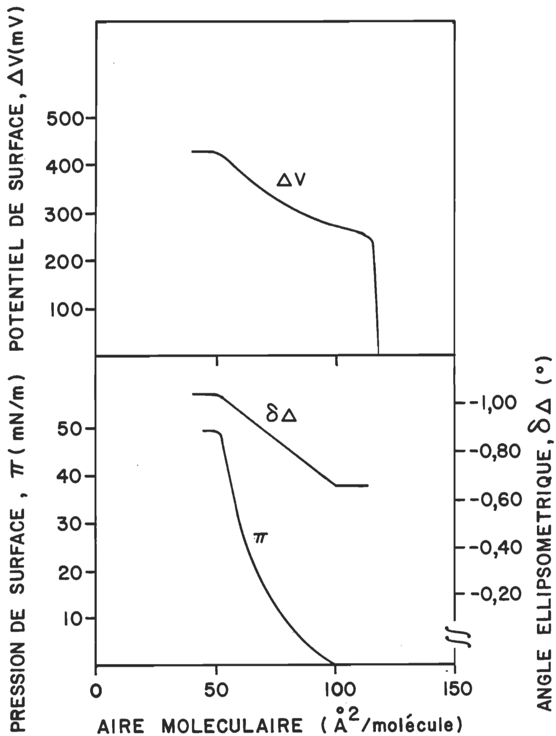
Figure 19. L'isotherme de pression, de potentiel de surface et ellipsoométrique de la POPC à l'interface azote-eau. La température est maintenue à 19,5 \pm 0,5^\circ\text{C} .
