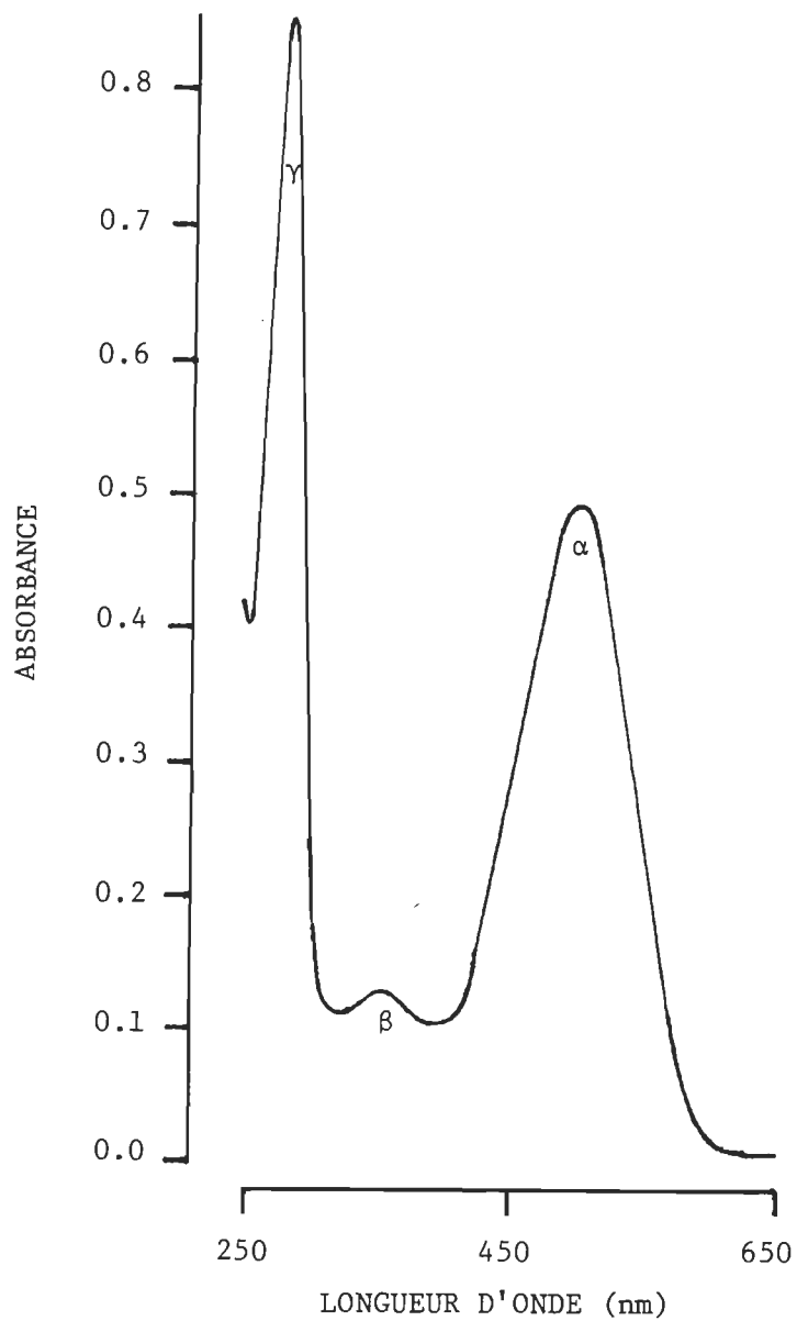
Figure III-3 : Spectre d'absorption électronique de rhodopsine purifiée solubilisée dans l'Ammonyx-L0. L'échantillon a été dialysé après la chromatographie d'affinité. La référence est un tampon Tris-Cl 50 mM pH 7.5 ajusté à 0.2% d'Ammonyx-L0. L'absorbance sur 2 mm est de 0.48 à 498 nm et de 0.84 à 278 nm. La pureté spectrale A_{278}/A_{498} est égale à 1.75. Le spectre de la rhodopsine présente les bandes \alpha , \beta et \gamma .
