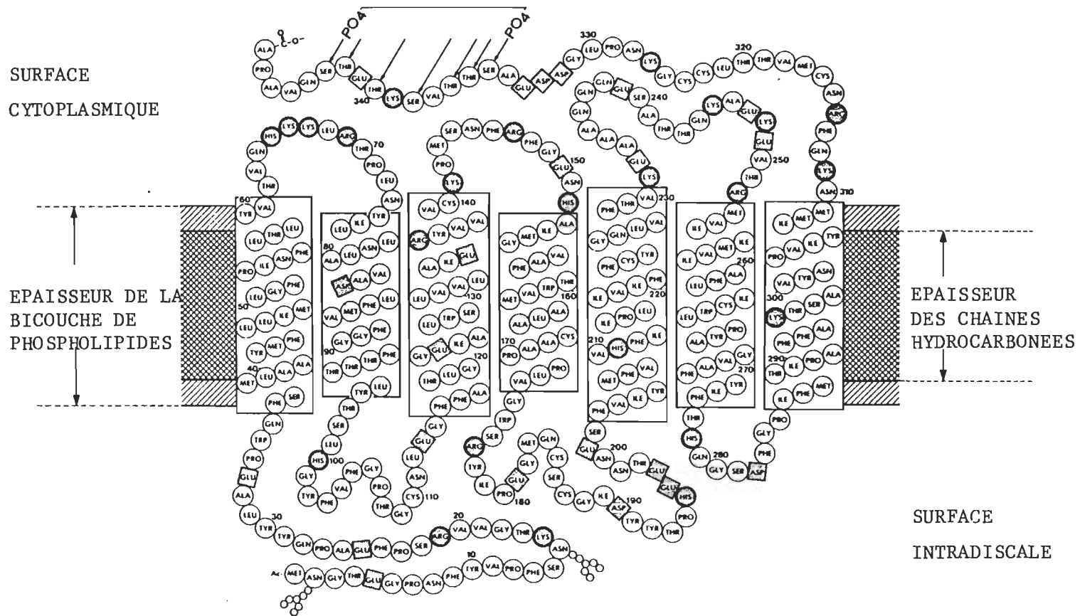
Figure I-3: Séquence des acides aminés de la rhodopsine bovine (Dratz et Hargrave, 1983). La rhodopsine est constituée de 348 acides aminés. L'extrémité carboxyle est exposée à la surface cytoplasmique du bâtonnet, tout comme les sites de phosphorylation indiqués par des flèches. Les acides aminés ayant des chaînes latérales chargées positivement sont représentés par des cercles ombrés. Les acides aminés à chaînes latérales chargées négativement sont indiqués par des carrés ombrés. Les hélices \alpha sont représentées par les rectangles perpendiculaires au plan de la membrane discale. L'extrémité aminée, à la surface intradisciale, porte les hydrates de carbone représentés par des chaînes de petits cercles.
