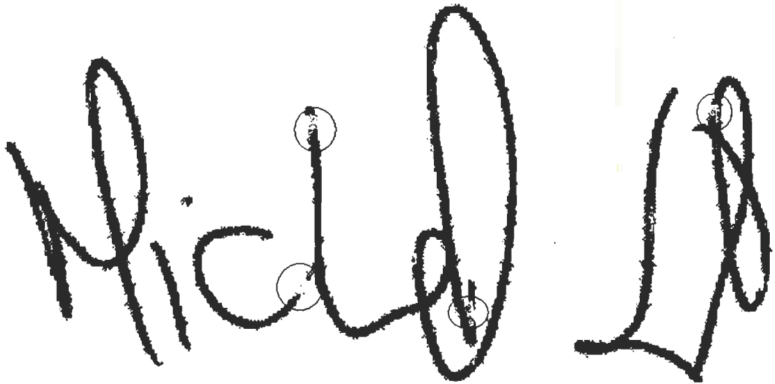
Figure 3.2 : Binarisation brut.
