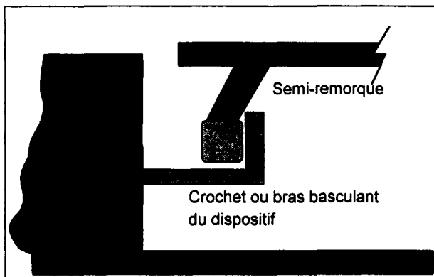
Figure 1. Dispositif à l'intérieur du quai
