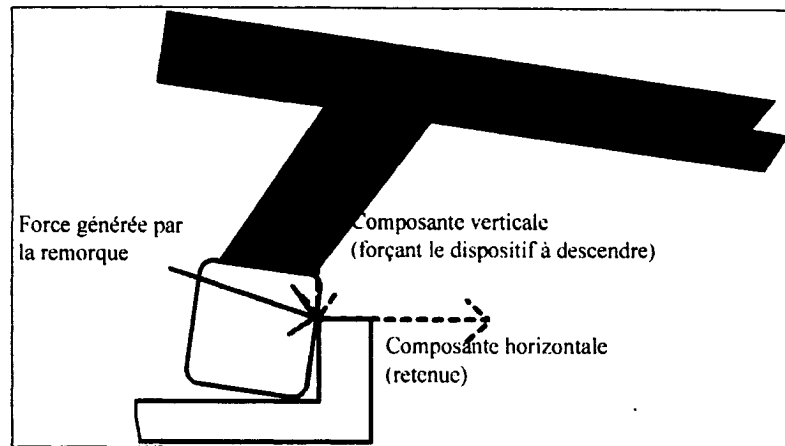
Figure 16. Angle de contact vers l'extérieur
