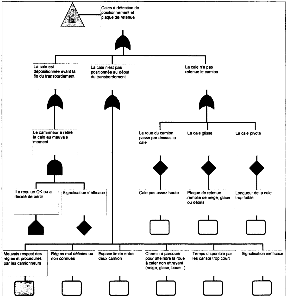
Figure 22. Mesure: cales à détection de positionnement et plaque de retenue
