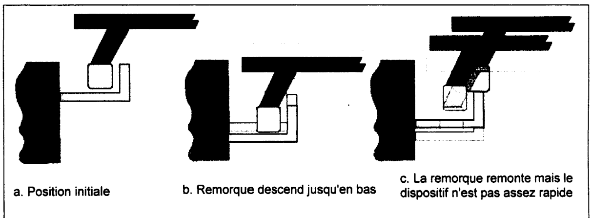
Figure 15. Décrochage de la barre anti-encastrement par un mouvement de suivi trop lent du dispositif
