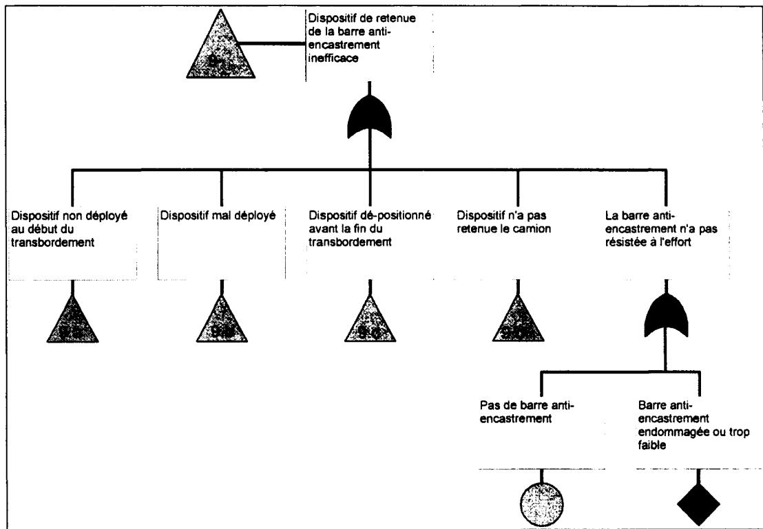
Figure 10. Mesure: dispositif de retenue de la barre anti-encastrement
