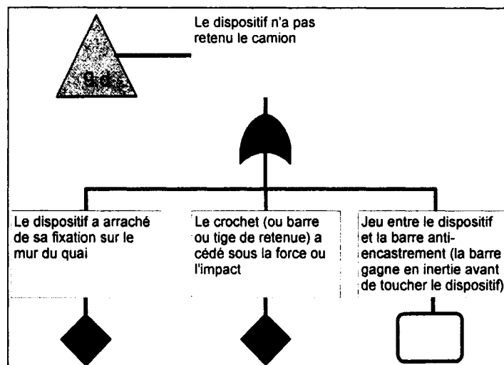
Figure 17. Mesure: dispositif de retenue de la barre anti-encastrement, n'a pas retenu le camion
