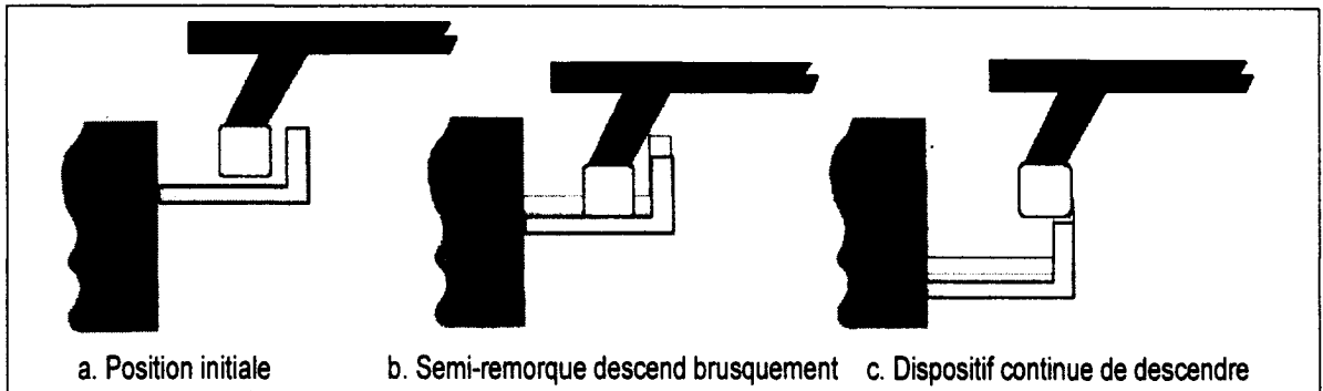
Figure 14. Décrochage de la barre anti-encastrement par un coup
