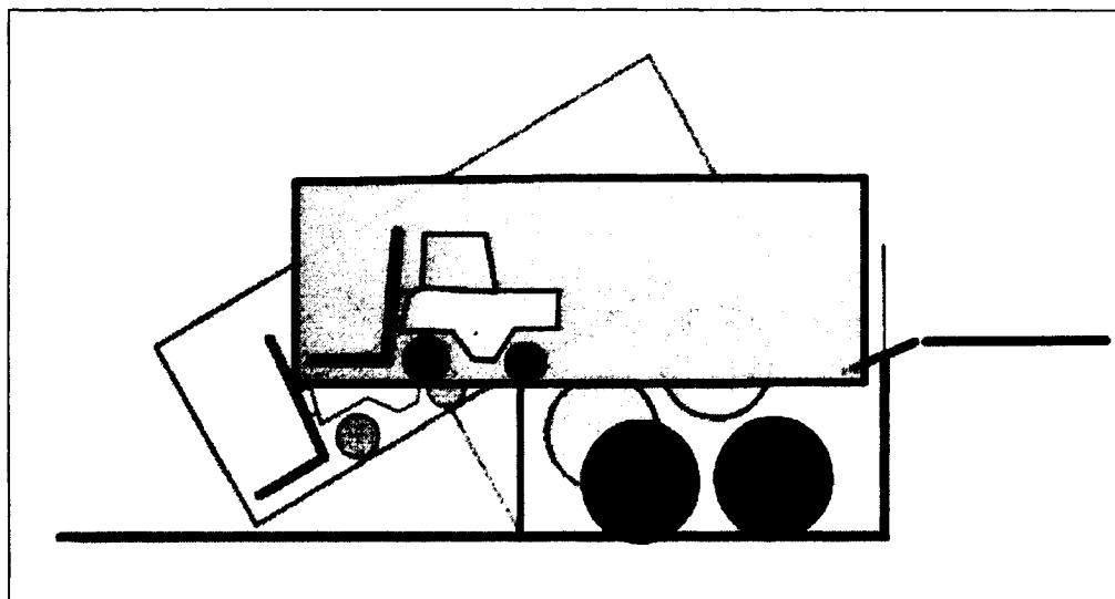
Figure 13: Situation à risque (semi-remorque courte)
