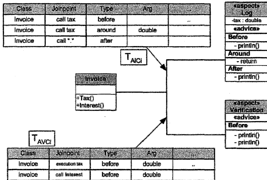
Figure 12 : Relation entre aspects et classes
