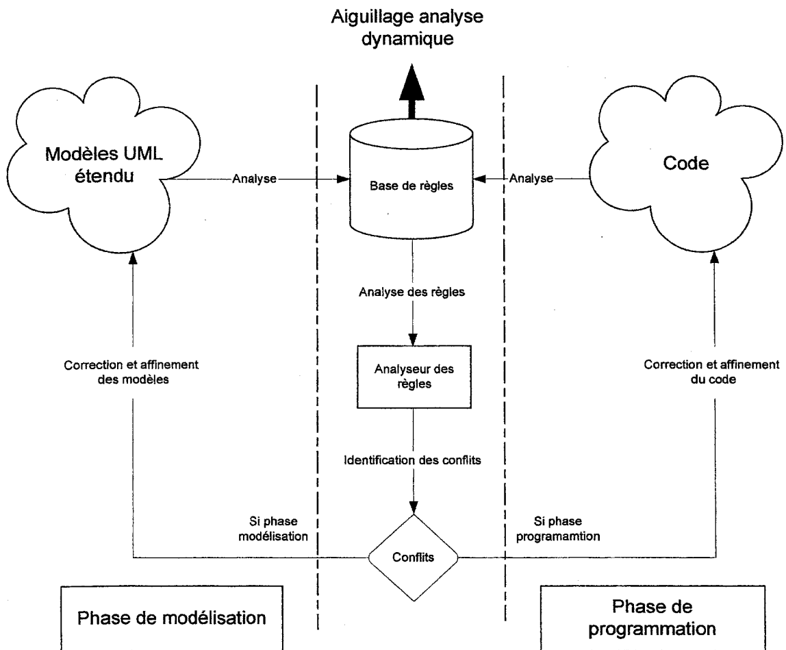
Figure 13 : Processus d'inférence
