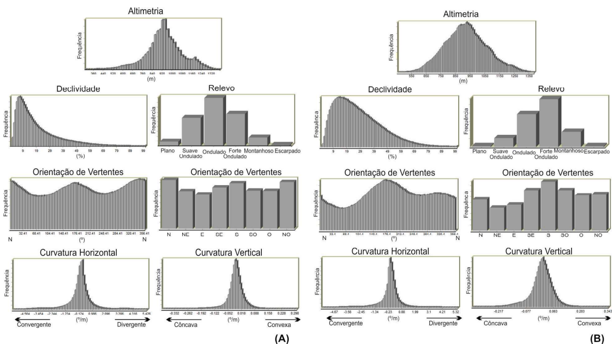
Fig. 4 - Distribuição de frequências de ocorrência das variáveis geomorfométricas em toda a área de estudo (A) e considerando apenas as regiões de FOM (B) mapeadas em 2010, na região nordeste do RS.
