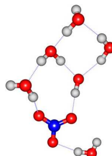
6wS 30 ; \Delta E = 7.67
