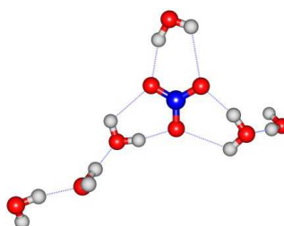
6wS 34 ; \Delta E = 8.53
