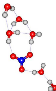
6wS 32 ; \Delta E = 8.13
