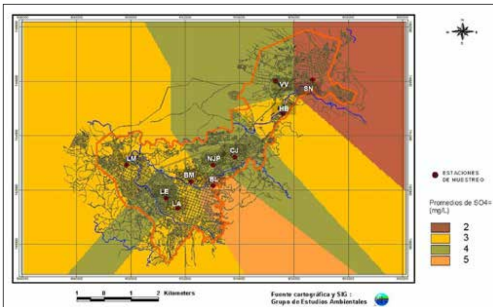
Figura 5. Distribución espacial y áreas de influencia directa e indirecta de \text{SO}_4^{2-} en el agua lluvia en la ciudad de Popayán.
