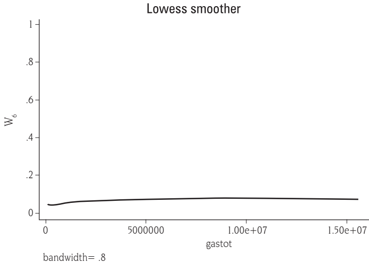
Gráfico 2. Curva de Engel para salud para Antioquia
