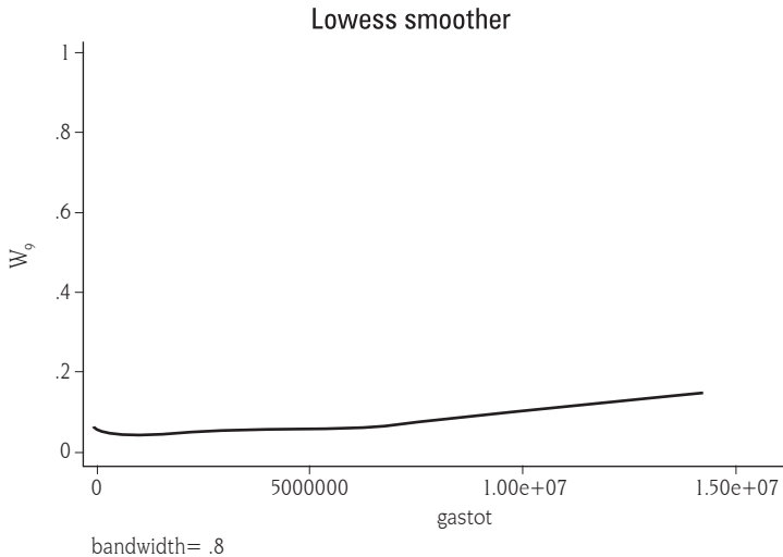
Gráfico 3. Curva de Engel para educación para Antioquia
