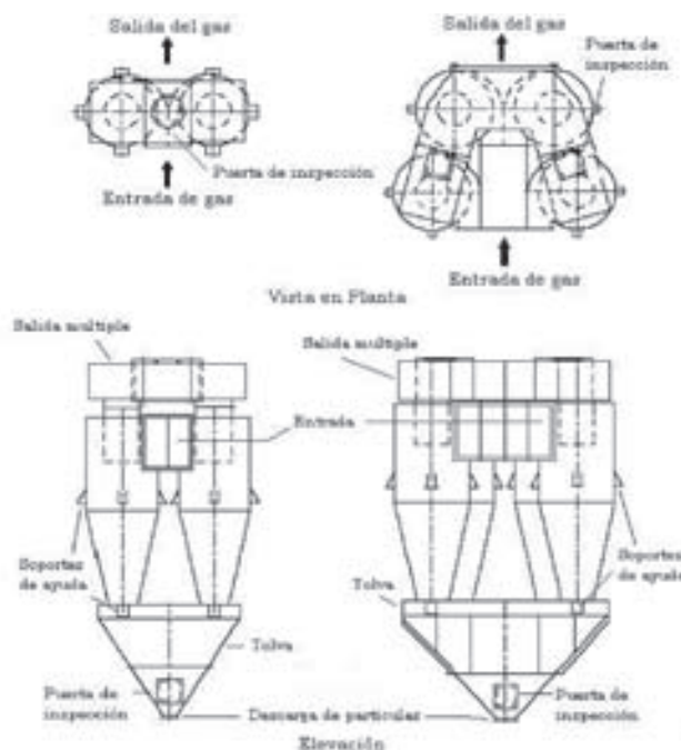
Figura 6. Multiciclones
