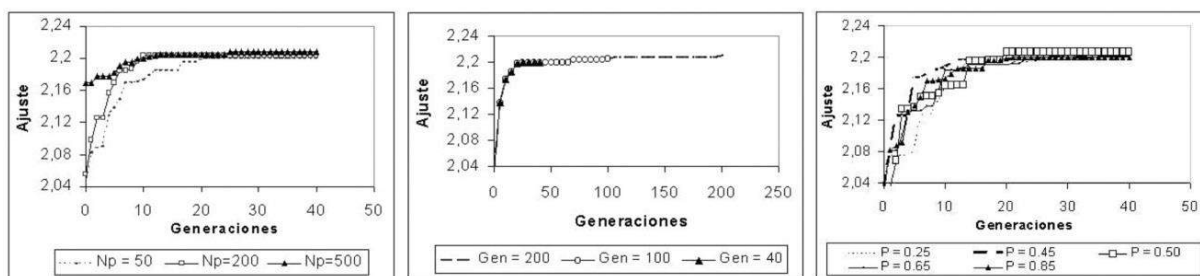
Figura 5. Ajuste de la función objetivo para diferentes tamaños de población, número de generación y probabilidad de cruce
