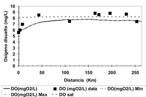
Figura 7. Validación del modelo QUAL2KW al río Sinú con los datos de campo
