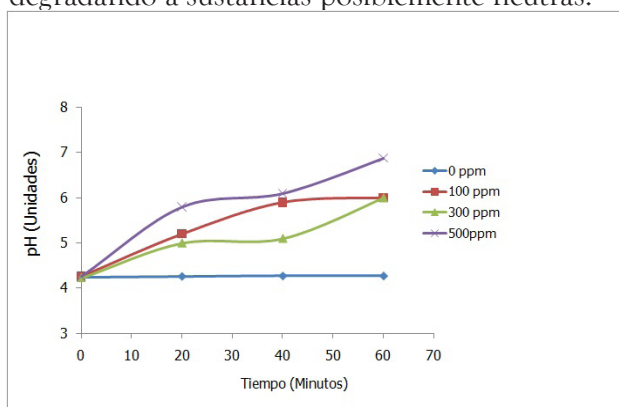
Figura 8. Variación del pH en el proceso fotocatalítico
