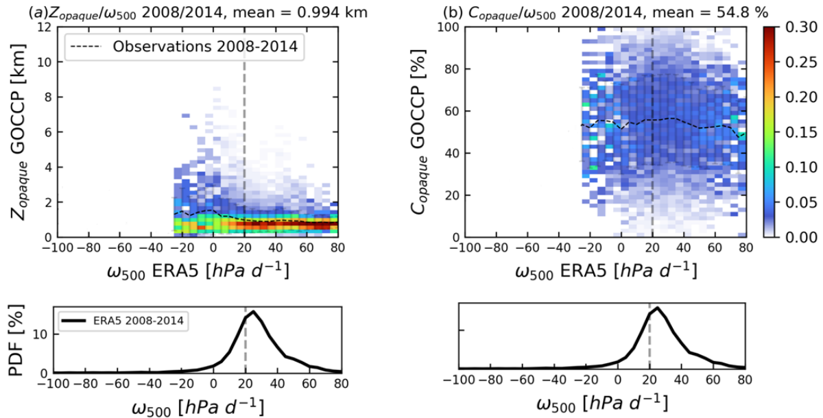
Figure 4.3 : Histogrammes normalisés montrant la distribution de (a) Zopaque [km] et la vitesse verticale du vent à 500 hPa \omega_{500} [hPa/d], et (b) Copaque [%] et \omega_{500} [hPa/d] en considérant les valeurs mensuelles moyennes sur une grille de 2^\circ \times 2^\circ dans la zone des stratocumulus au bord de la côte ouest Africaine [27°S/6°S-80°O/110°O], au dessus des océans uniquement, pour la période 2008-2014. Sous chaque histogramme normalisé se trouve la PDF de \omega_{500} [hPa/d] sur la période 2008-2014. Zopaque et Copaque proviennent des observations CALIPSO-GOCCP, \omega_{500} des réanalyses ERA5. La ligne verticale en pointillés représente \omega_{500} = +20 hPa/d (voir texte). Les plages de \omega_{500} contenant moins de 40 occurrences sont masquées (blanc). La résolution des données est de 2^\circ \times 2^\circ \times 1 mois.
