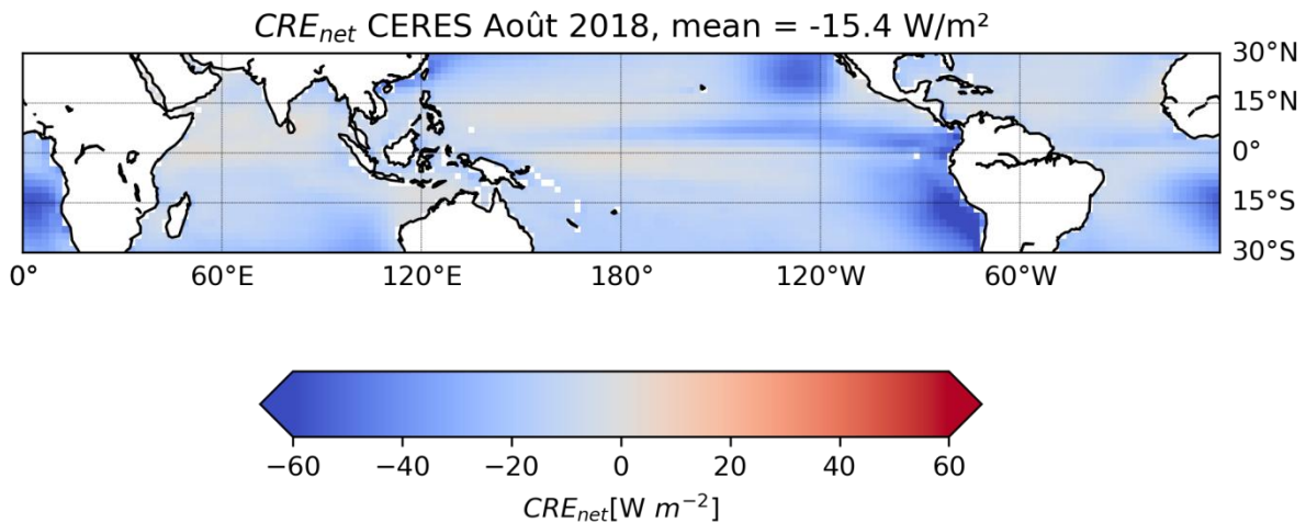
Figure 3.5 : Carte de CRE_{net} issue des observations CERES moyenné sur le mois d'août 2018 regriddée à la résolution GOCCP. Le rouge représente un CRE_{net} positif et le bleu représente un CRE_{net} négatif.
