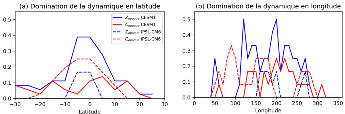
Figure 5.15 : PDF de la domination de la dynamique suivant (a) une coupe latitudinale et (b) longitudinale. La courbe bleue représente Z_{opaque} et la courbe rouge C_{opaque} (courbe pleine pour CESM1 et courbe pointillée pour IPSL-CM6).
