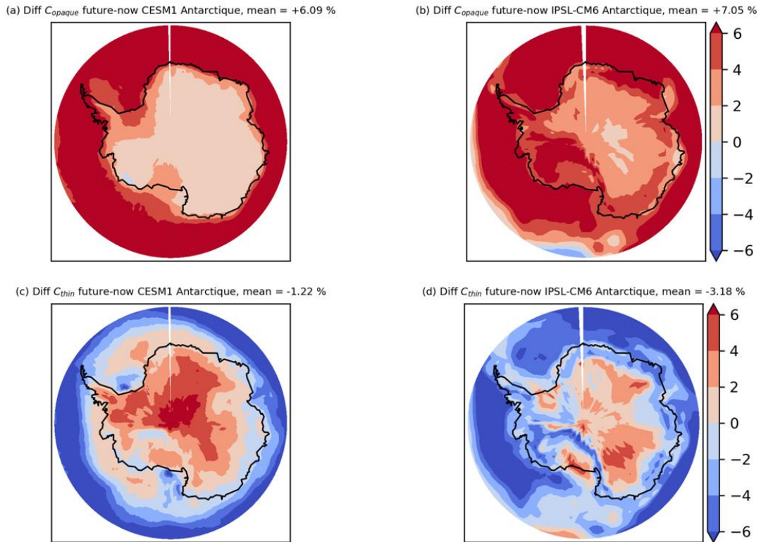
Figure 7.2 : Cartes de différence entre le futur (2083-2095) et le présent (2008-2020) de la couverture en (a et b) nuages opaques (Copaque) et (c et d) nuages fins (Cthin). La colonne de gauche fait référence au modèle CESM1 et la colonne de droite au modèle IPSL-CM6.
