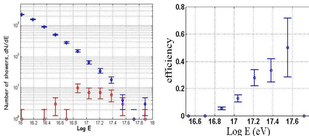
Figure 19.: A gauche : distribution de l'énergie mesurée par le détecteur de particules (points bleus) et des événements détectés en radio pour les événements internes dont le coeur est localisé dans un rayon de 200 m autour du centre du réseau. A droite : efficacité de détection de la radio en fonction du log de l'énergie de la gerbe (exprimée en eV).
